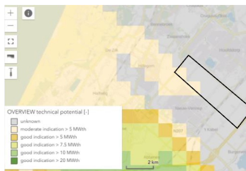
Figuur 4.6: Geothermie potentie
