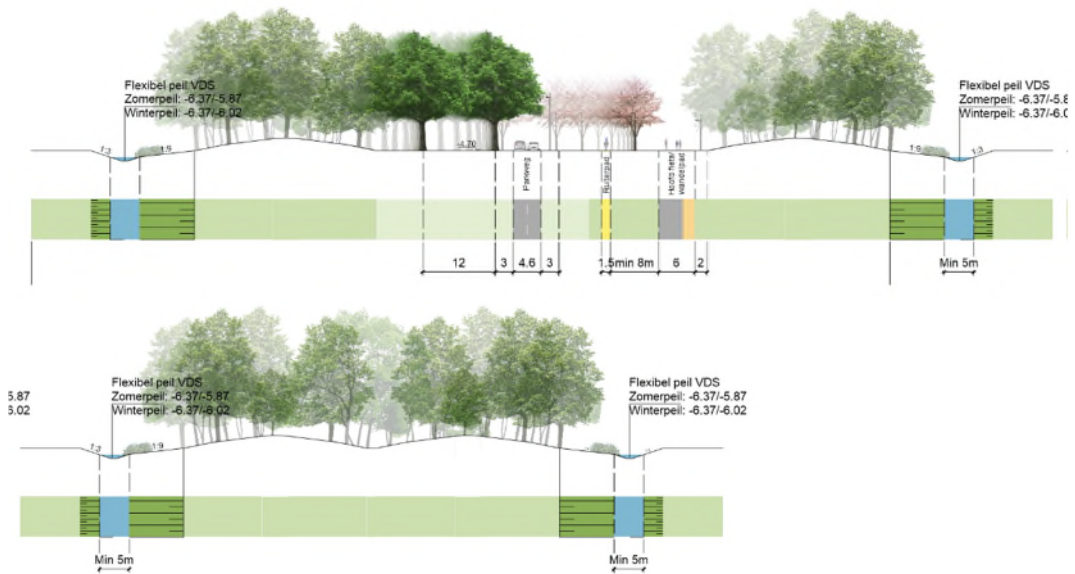
Figuur 4.1: Principe oplossing voor dwarsdoorsnedes prioritaire structuur (parklaag)
