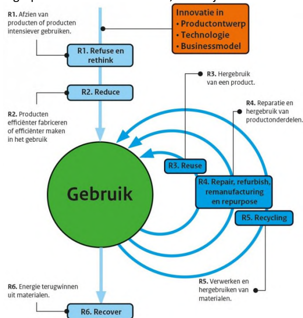
Figuur 13.1: Circulariteitsladder
