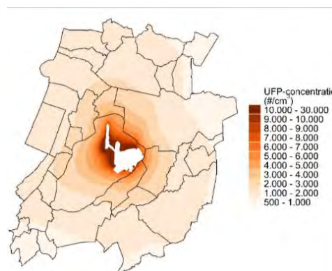
Figuur 4: Gemiddelde gemodelleerde concentratie UFP van vliegverkeer voor de periode 2006-2019 in het onderzoeksgebied. Het terrein van Schiphol is wit, omdat daar geen mensen wonen (Bron: RIVM ).
