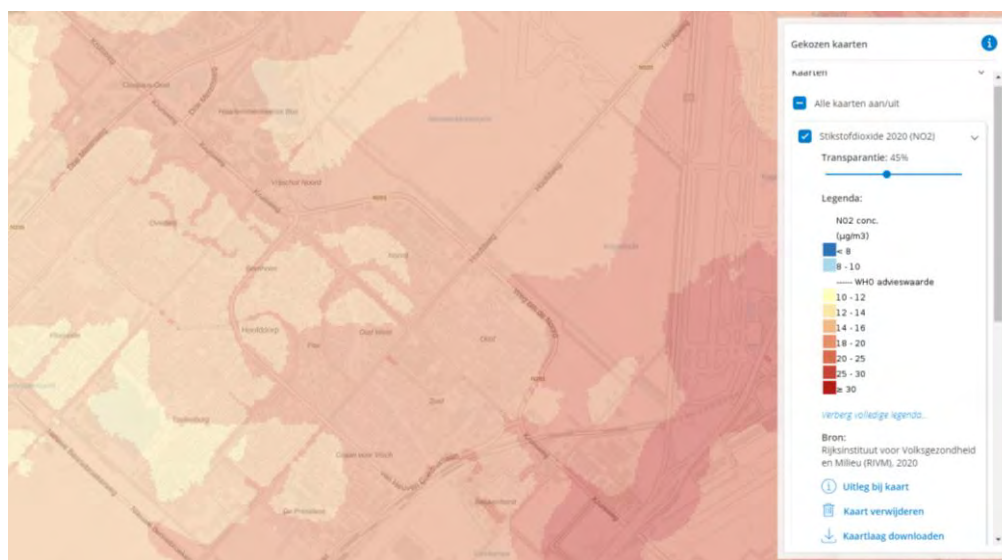
Figuur 3: Stikstofdioxide 2020 ( \text{NO}_2 ) in Hoofddorp Noord (bron: Kaarten | Atlas Leefomgeving )
