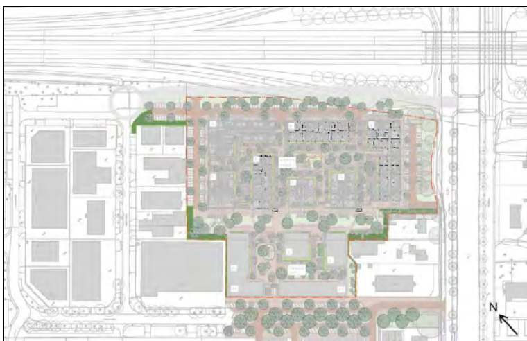
Figuur 1 - situatietekening
