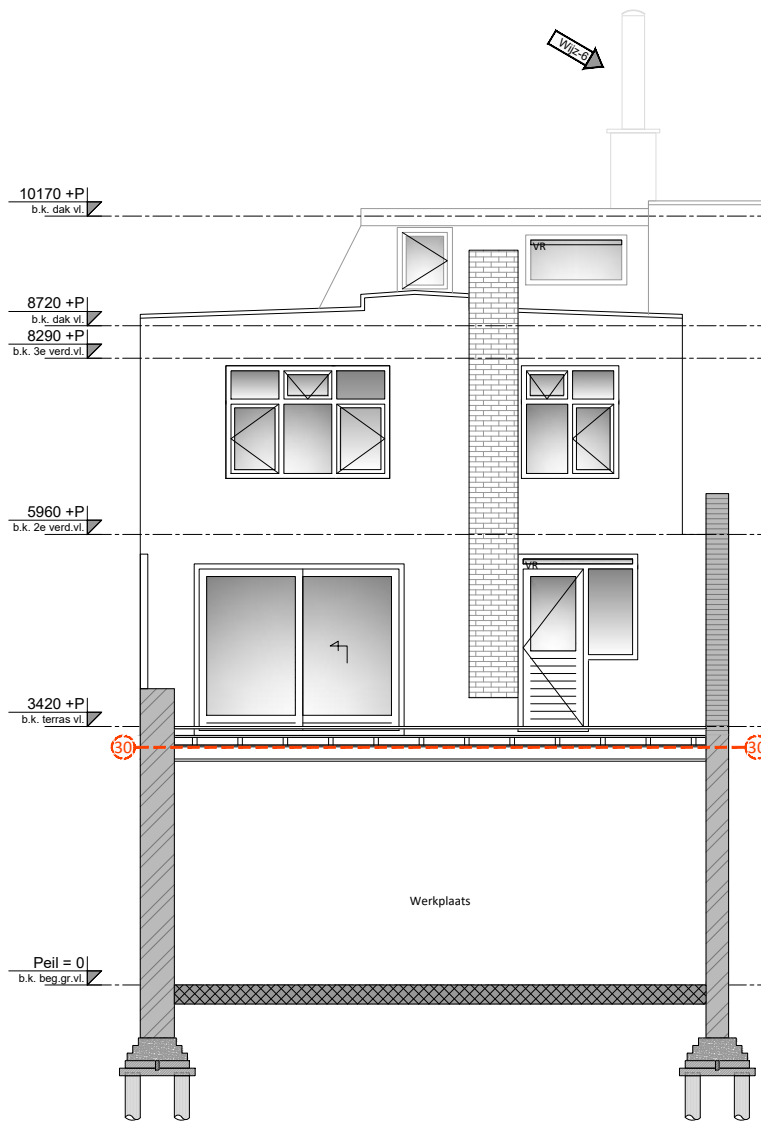
ACHTERGEVEL Bestaande situatie
