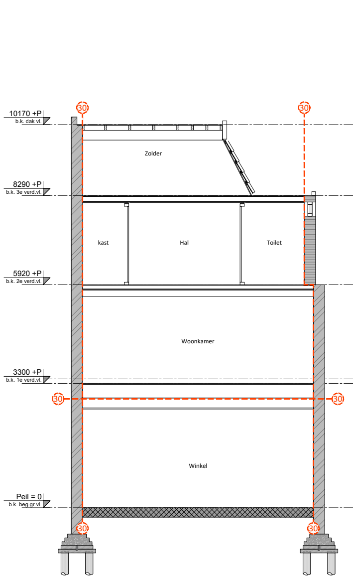
DOORSNEDE B-B Bestaande situatie
