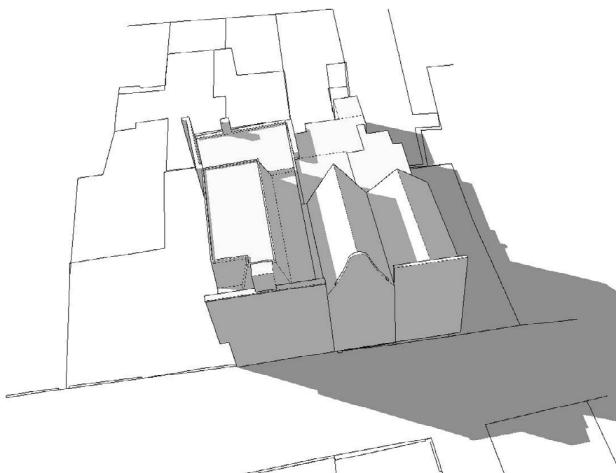
bestaand voorgevel 21 maart 15.00 uur
