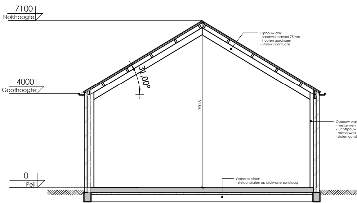
Doorsnede A-A
