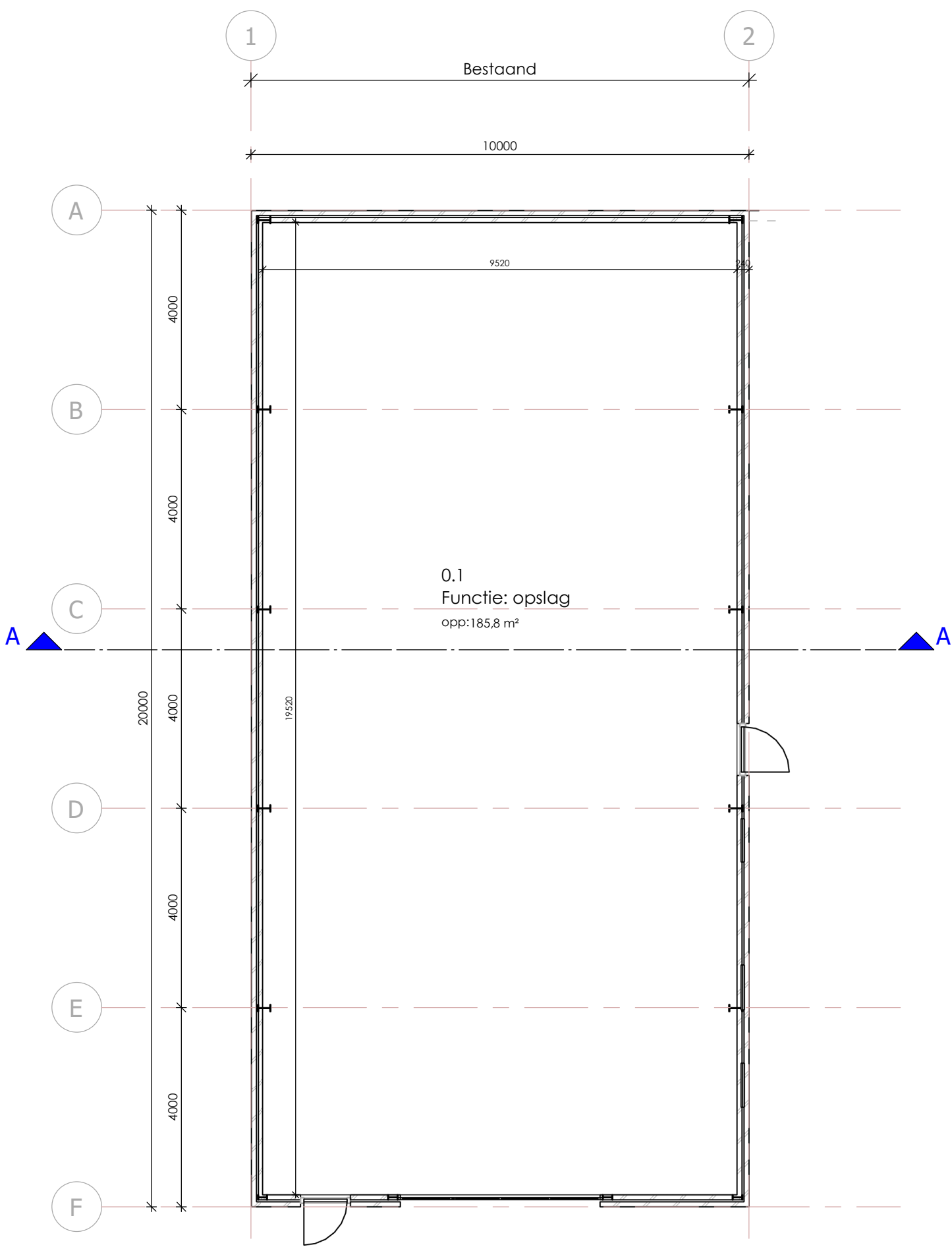
Begane grond
