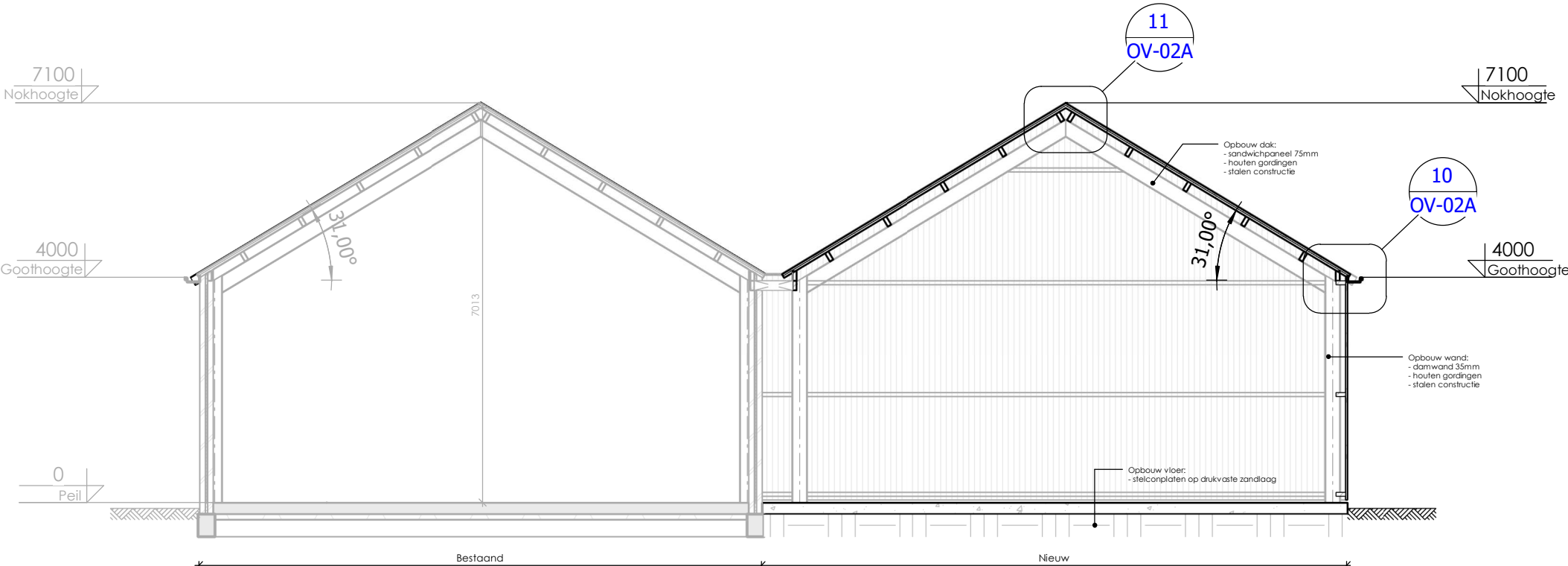
Doorsnede A-A
