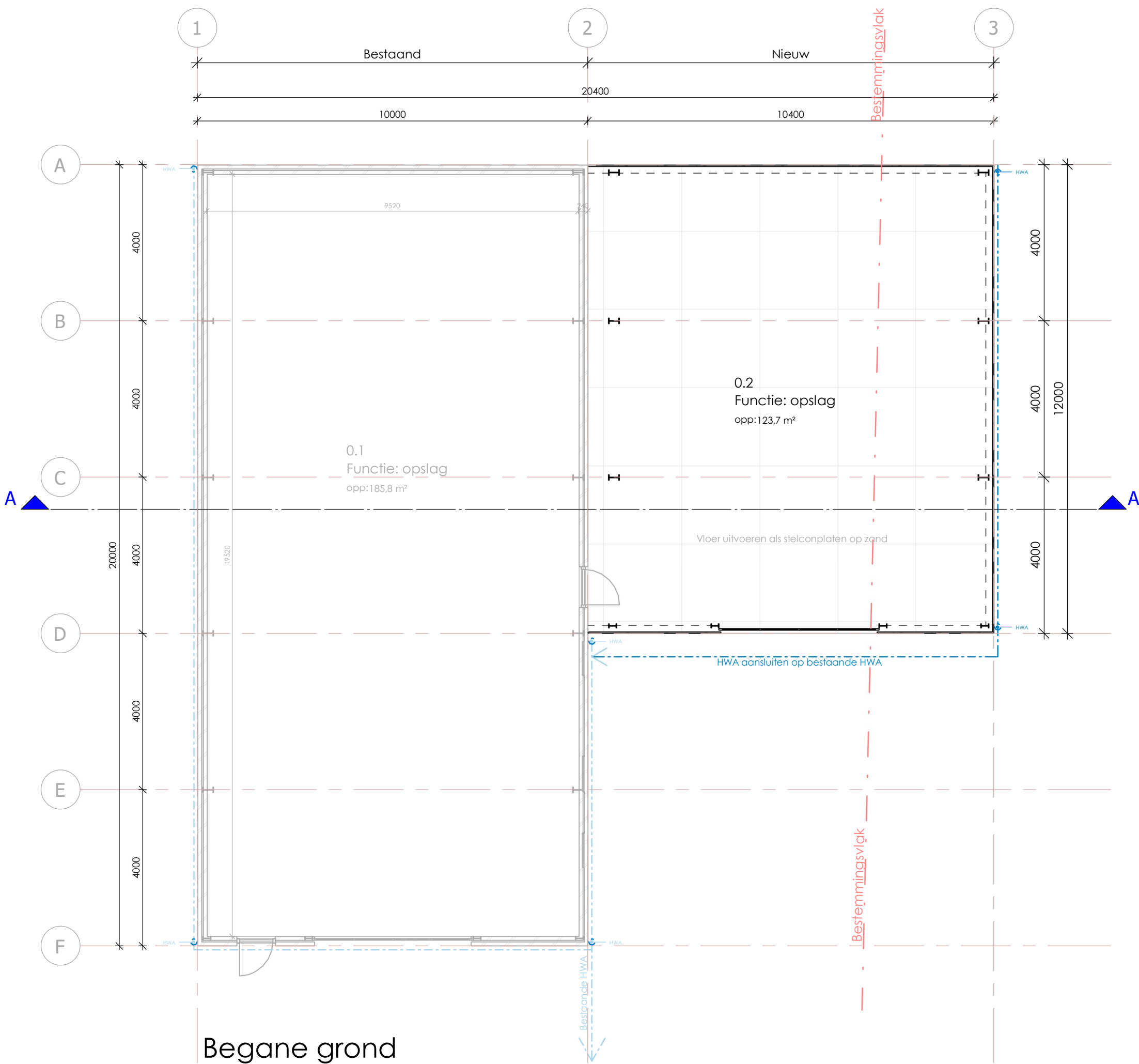
Begane grond
