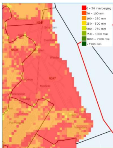
Figuur 23.3 Waterbergend vermogen van de ondergrond (Leefomgevingsfoto, 2020)
