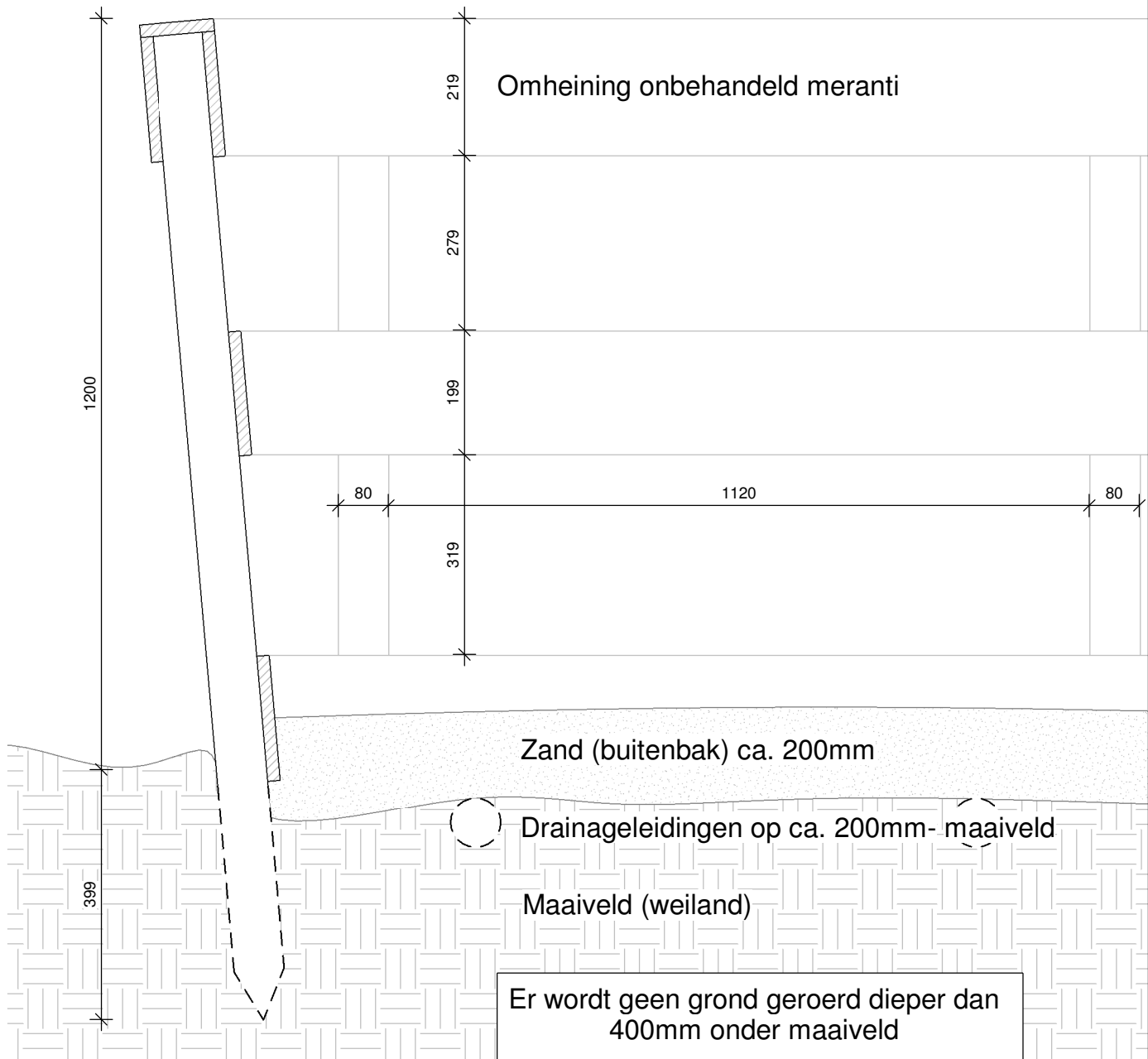
Principedetail buitenbak / paddock
