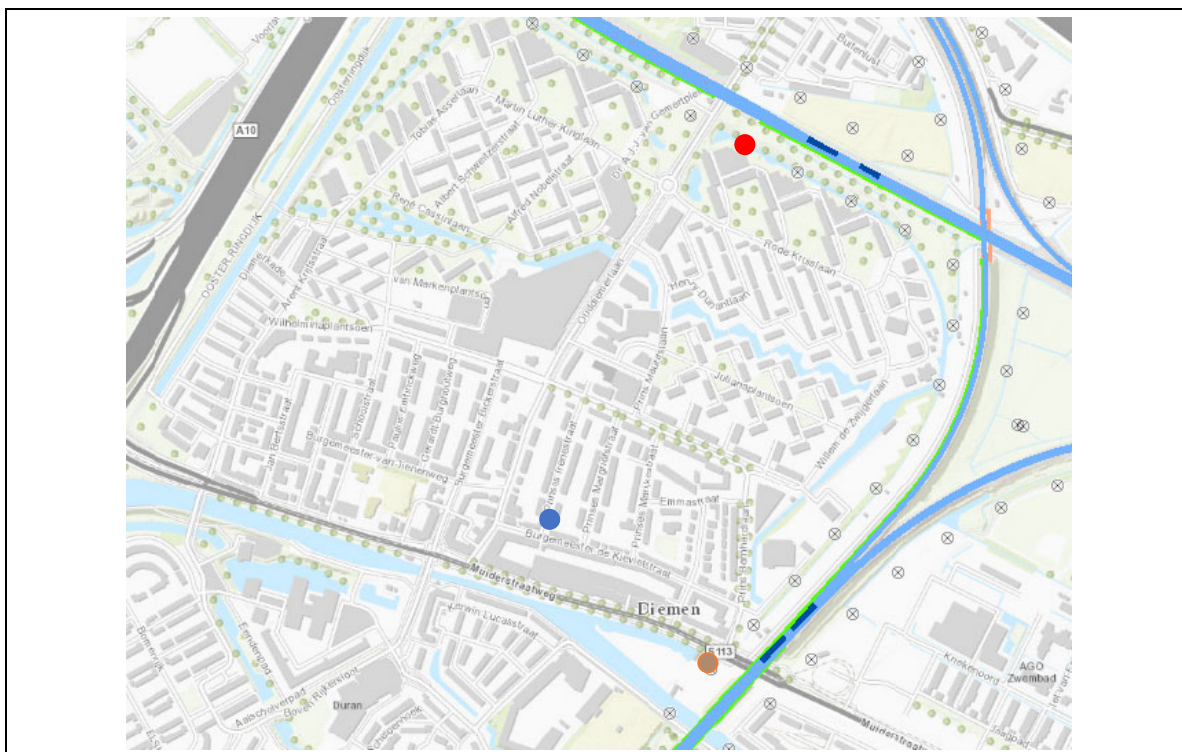
Figuur 2.1: Maatgevende geluidproductieplafonds 62,4 dB (rode stip) en 57,1 dB (bruine stip). Locatie nieuwe woning blauwe stip
