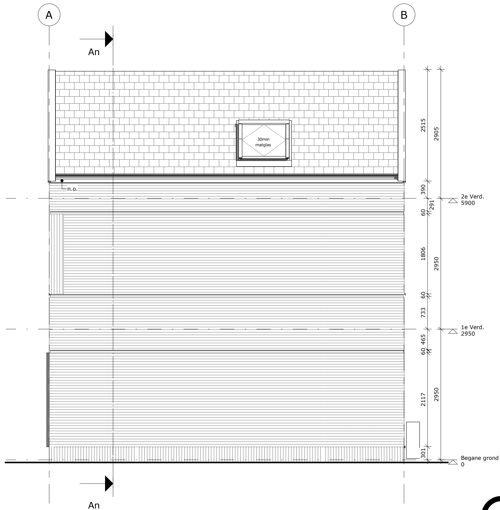
Rechter gevel (noord)
