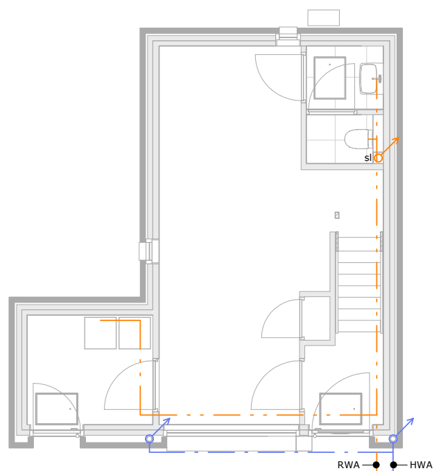
Begane grond
