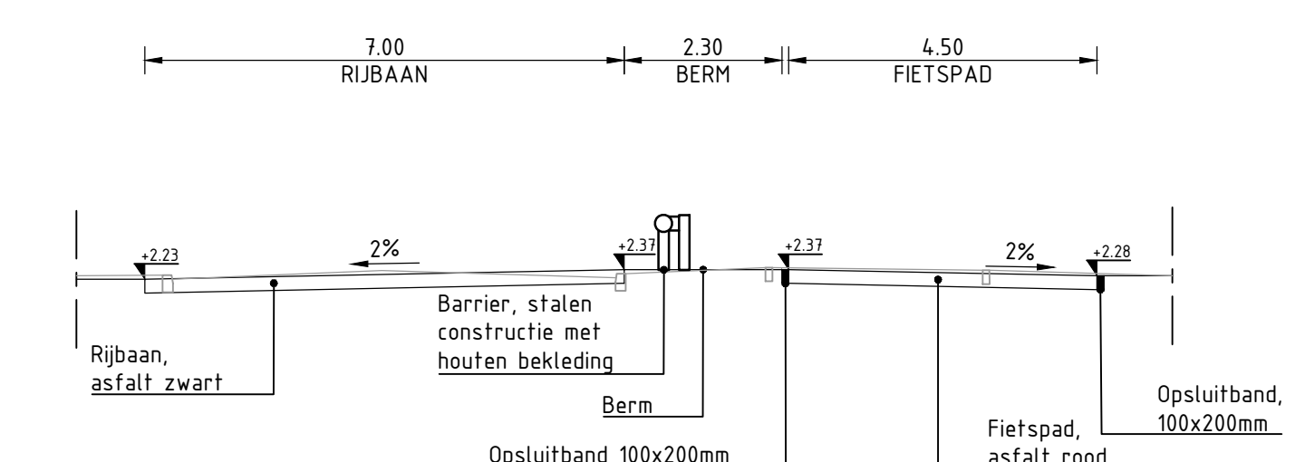
DWARSPROFIEL B-B'
