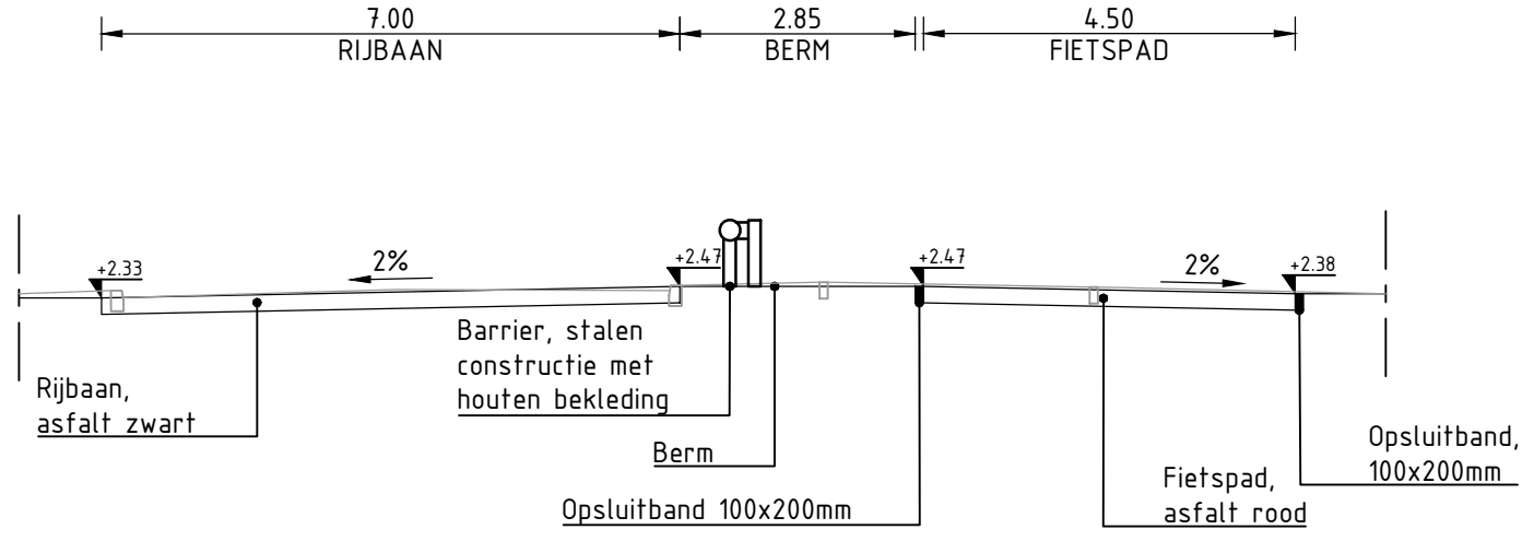
DWARSPROFIEL C-C' Schaal 1:100
