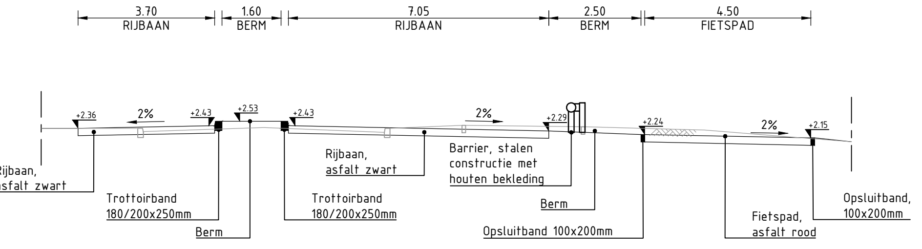
DWARSPROFIEL A-A'
