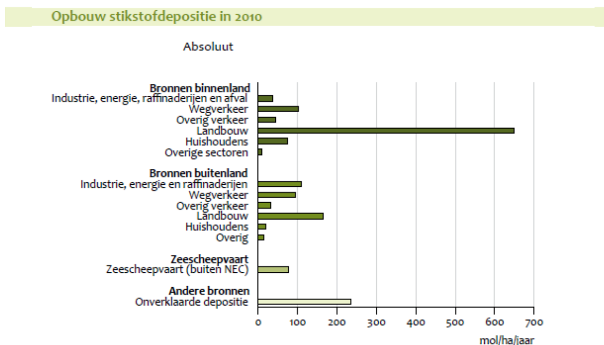
Figuur 8 Herkomst van de stikstofdepositie (bron: Planbureau voor de leefomgeving, 2010)
