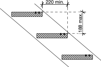
Principe trap
