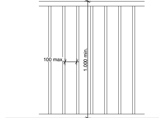
Principe balustrade
