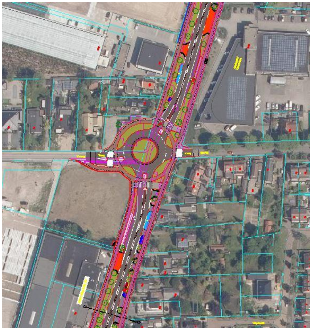
Afbeelding 3.1: Realisatie rotonde Rijksweg - Visweg
