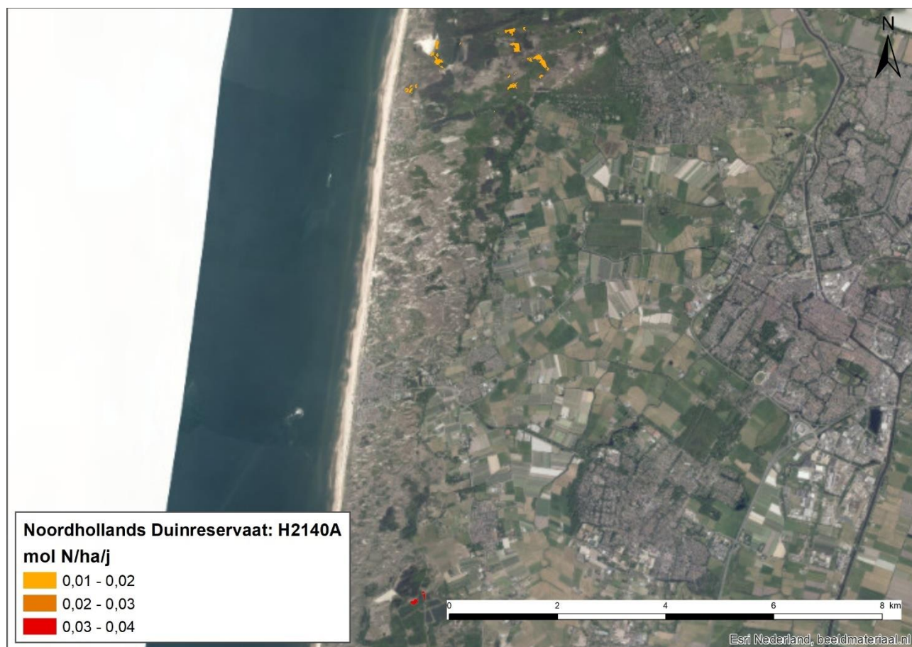
Figuur 9 Toename stikstofdepositie als gevolg van de aanleg van de Aansluiting A9 Heiloo op locaties met habitattype H2140A Duinheiden met kraaihei (vochtig) met overschrijding van de KDW. Noordhollands Duinreservaat
