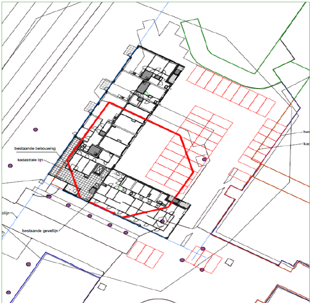
Ligging van de huidige bebouwing (rode lijn), nieuwe parkeervoorzieningen (dunne rode lijnen) en nieuwe bebouwing (zwart ingetekend).
