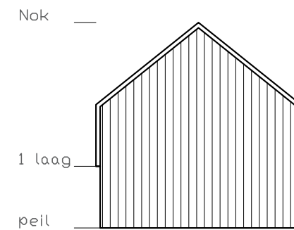
Dakbedekking doortrekken langs gevel tot laag 1
