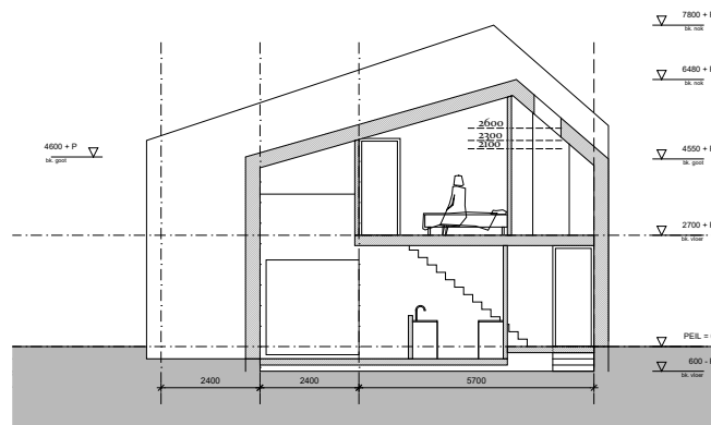
doorsnede 3
