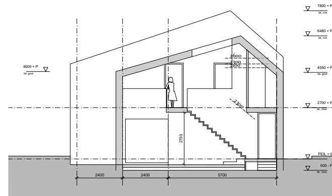
doorsnede 2
