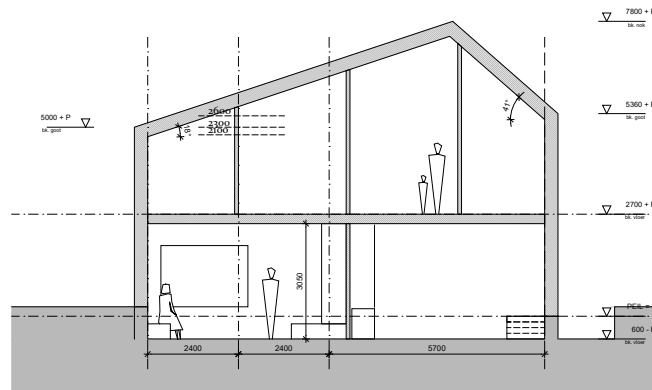
doorsnede 1
