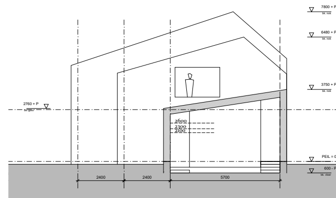
doorsnede 4
