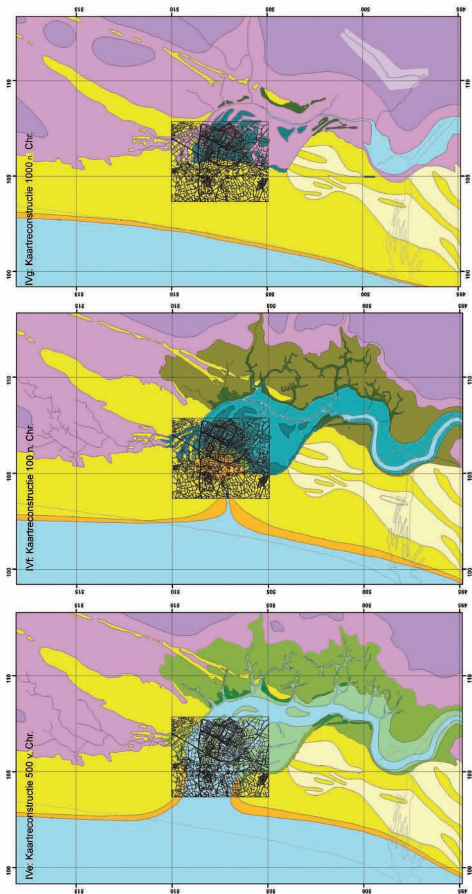
Afbeelding 6: De huidige ligging van Castricum en het plangebied (in rood) geplot op de loop van en de situatie rond het Oer-IJ in 500 v. Chr., 100 AD en 1000 AD. Zie voor legenda afbeeldingen 4 en 5.
