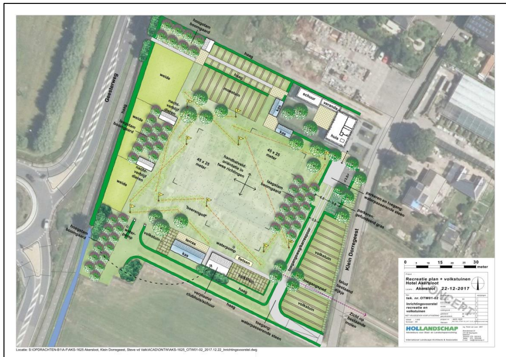
Inrichtingsvoorstel voor het plangebied.
