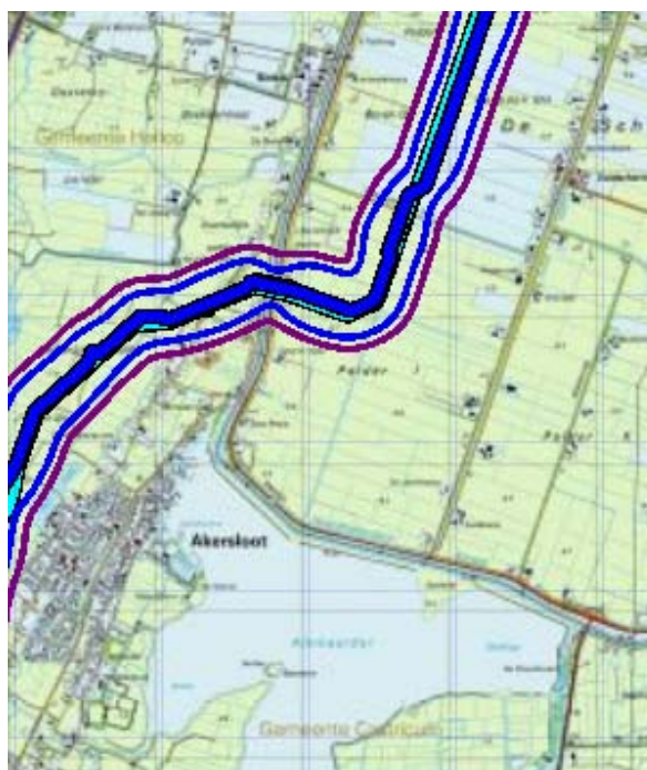
Figuur 4.4 Plaatsgebonden risico voor A-620
