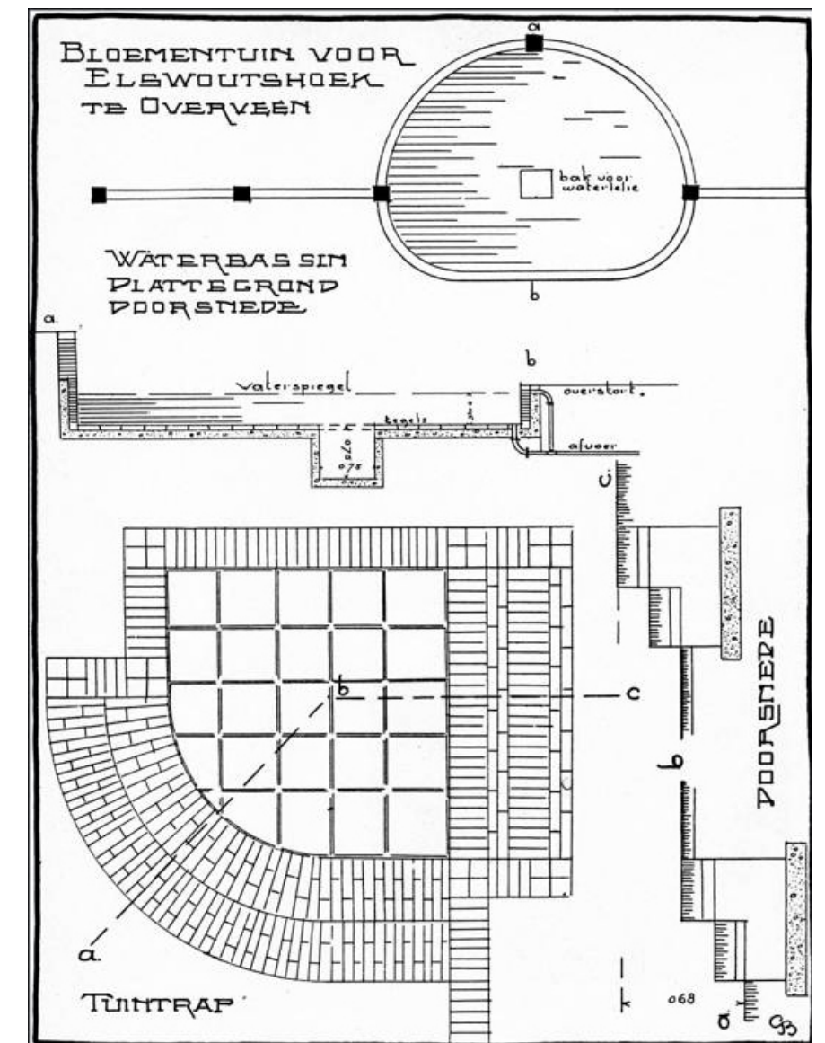
Bloementuin van G. Bleeker, waterbassin en tuintrap, constructietekening. Uit: G. Bleeker, Tuinkunst (ca. 1950)
