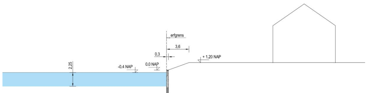
doorsnede en peilen
