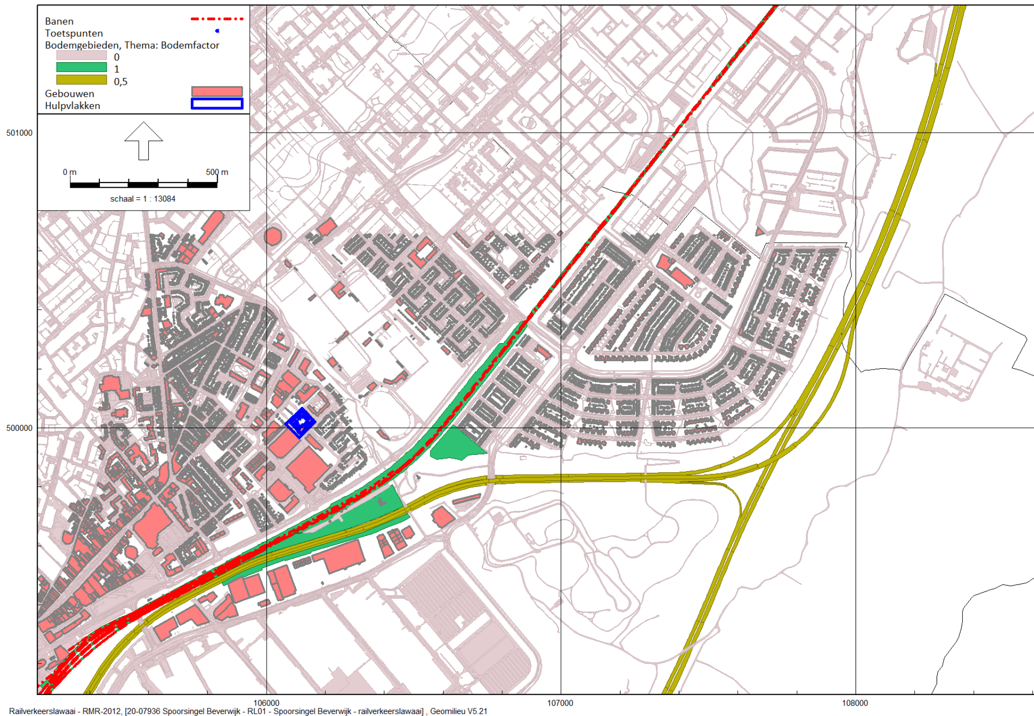
Figuur 6 | Overzicht rekenmodel railverkeerslawai
