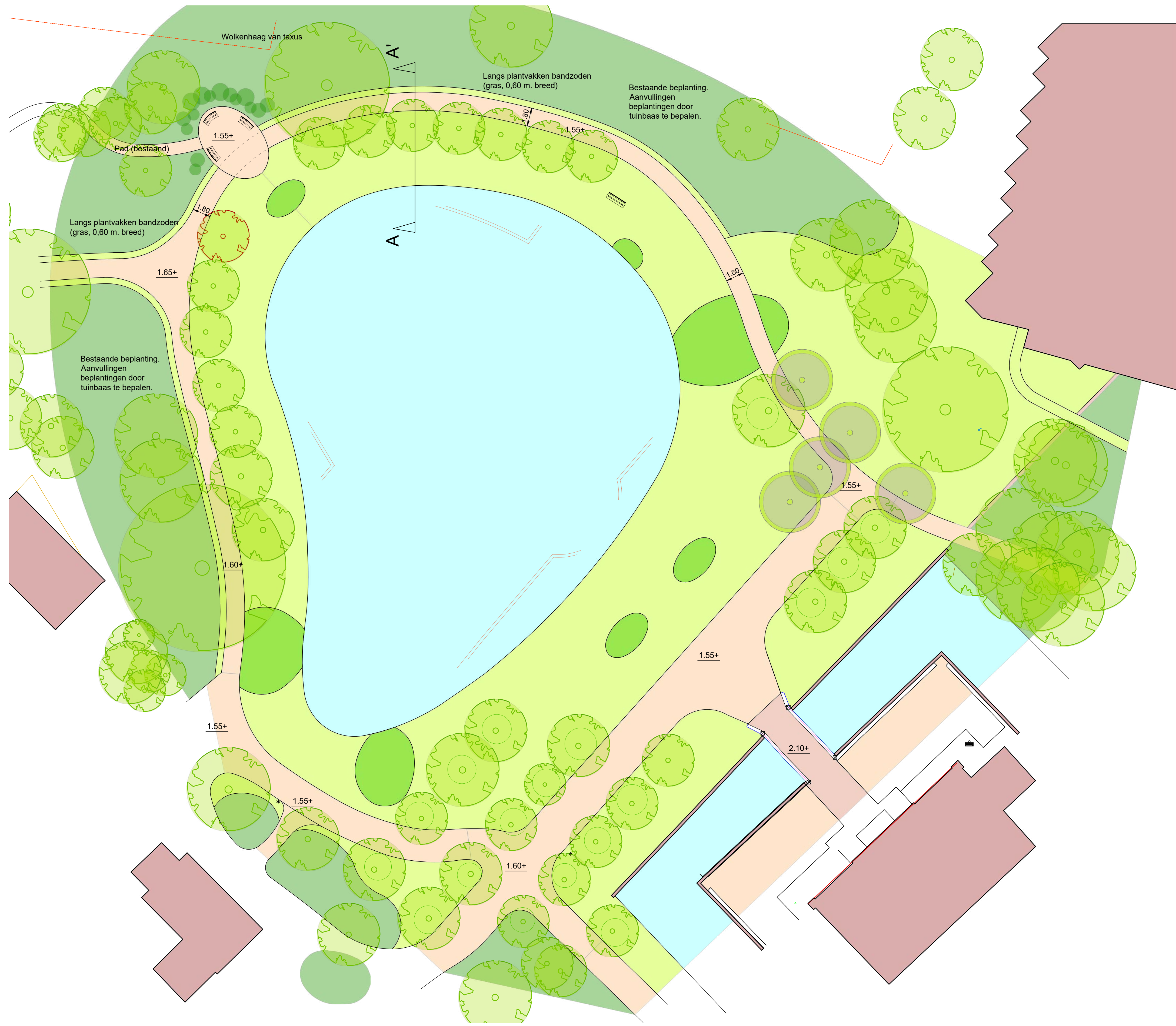
Definitief Ontwerp 1 : 200
