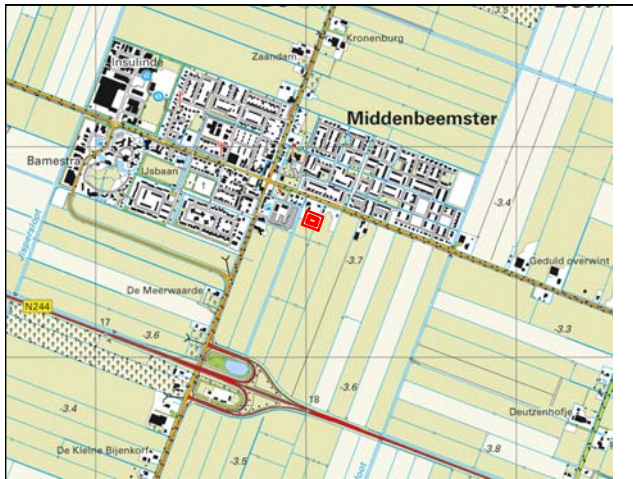
Overzichtskartaal
