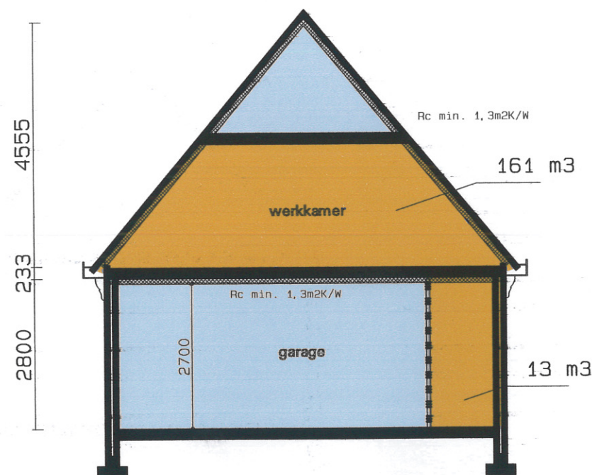
doorsnede B-B
