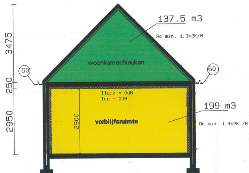
doorsnede A-A
