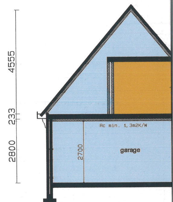
doorsnede C-C
