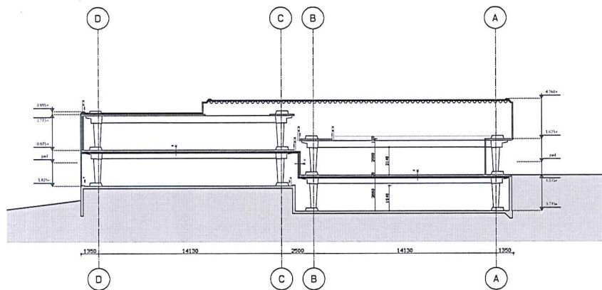
Doorsnede EE
