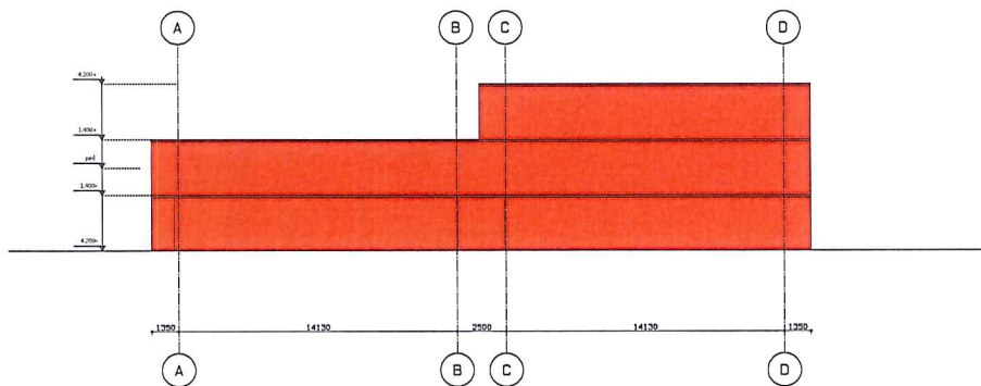
Zuidgevel
