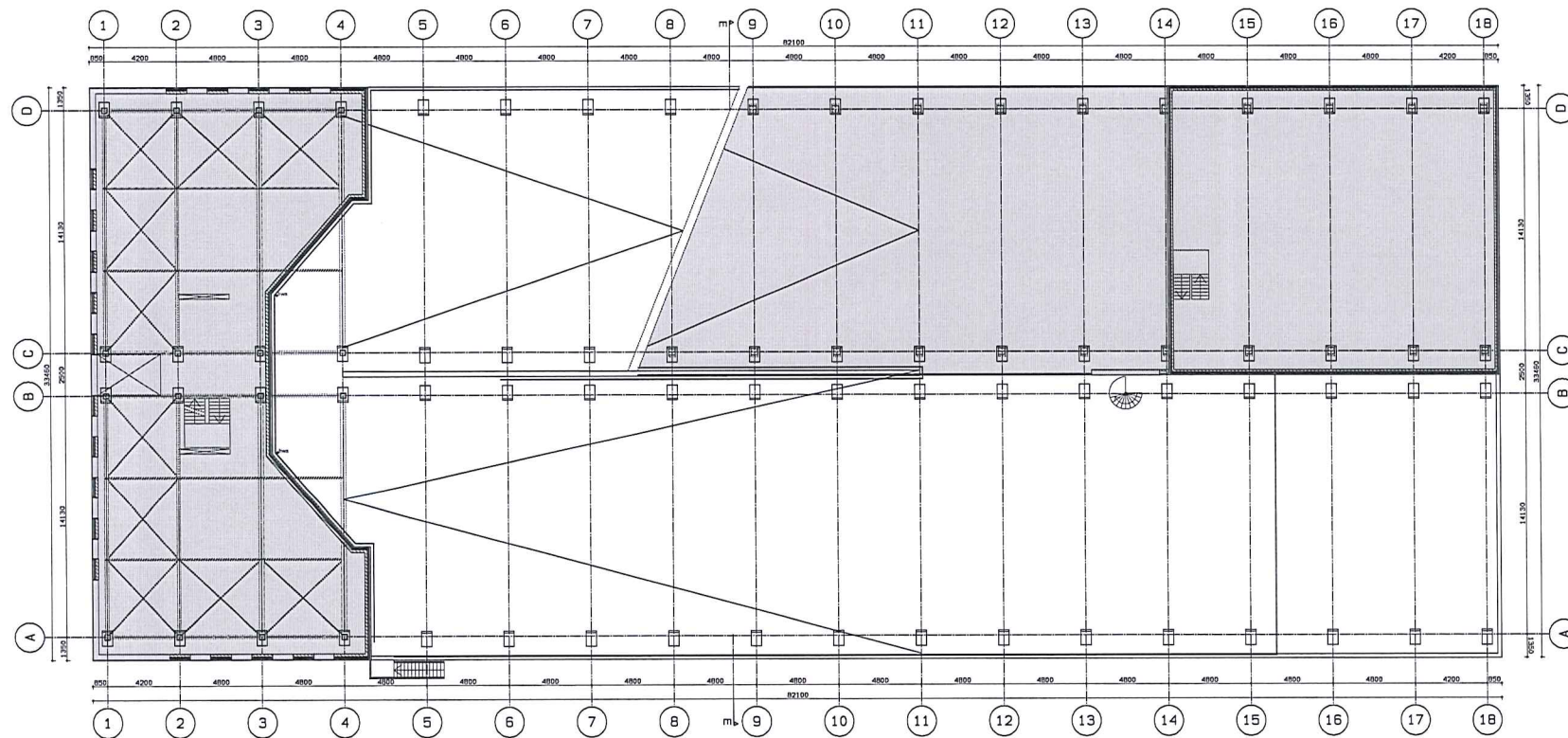
laag 3
