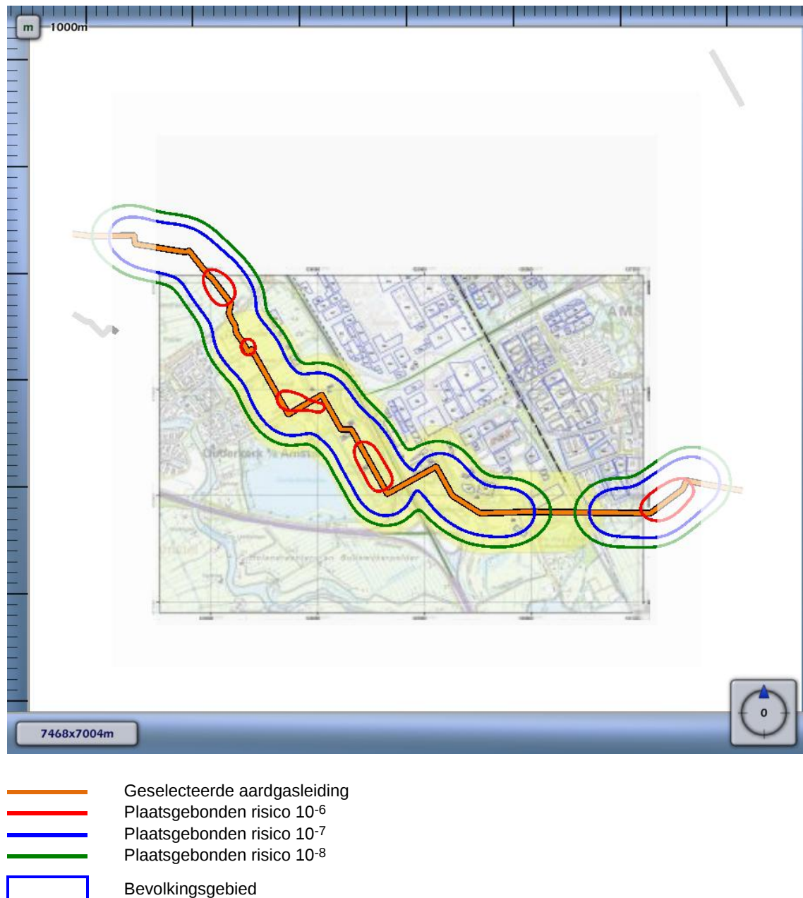
Figuur 3.1 Plaatsgebonden risico voor W-534-39 van N.V. Nederlandse Gasunie
