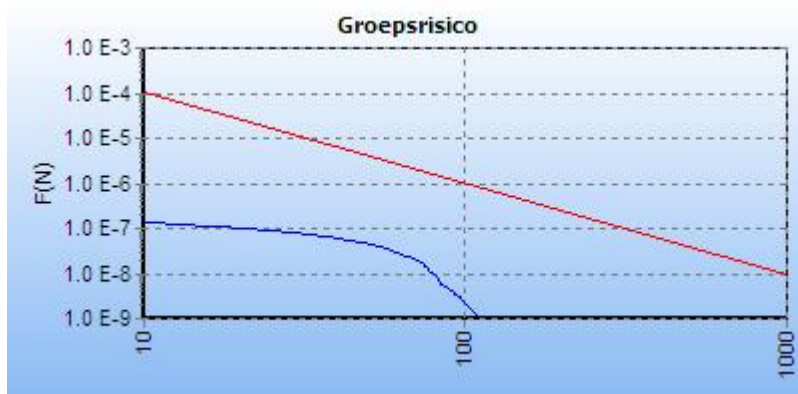
Figuur 5.1 FN curve voor W-534-39 van N.V. Nederlandse Gasunie voor de kilometer tussen stationing 13350.00 en stationing 14350.00
