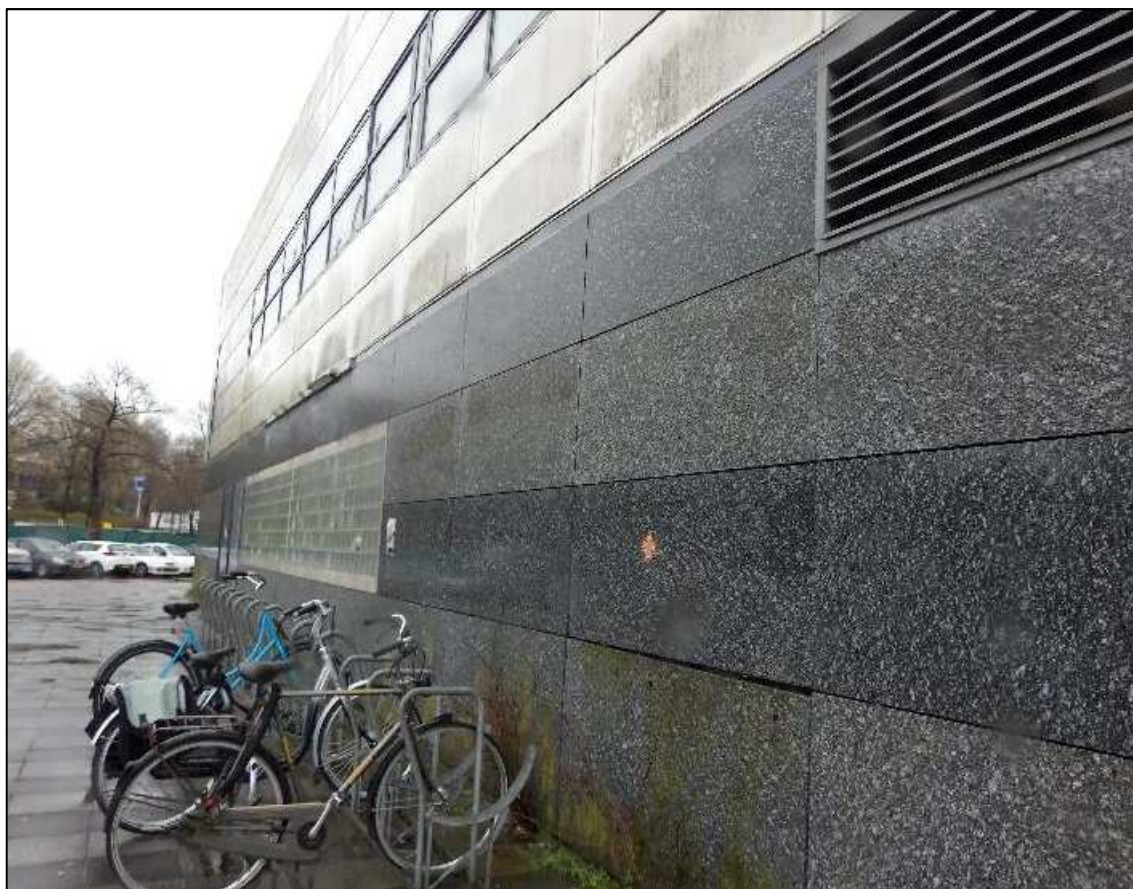
De openingen tussen de beplating van de bebouwing zijn afgesloten en lopen niet door naar een geschikte achterliggende ruimte. Ook zijn de panelen erg glad.
