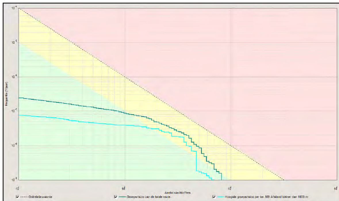
Figuur 3.3 FN curve groepsrisico bestaande situatie.
