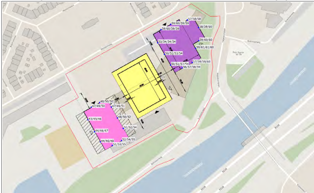
f5 Gecumuleerde geluidbelasting alle wegen samen (in dB Lden exclusief en inclusief aftrek conform art. 110g Wgh).
