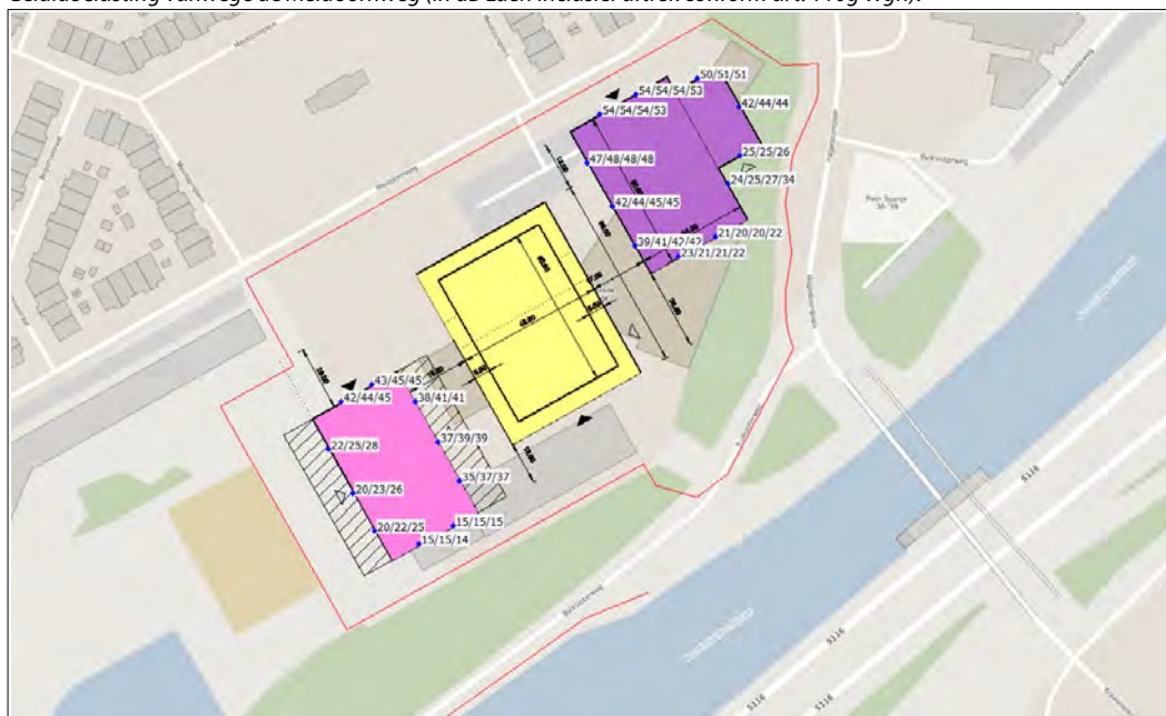
f4 Geluidbelasting vanwege de Meidoornweg (in dB Lden inclusief aftrek conform art. 110g Wgh).
