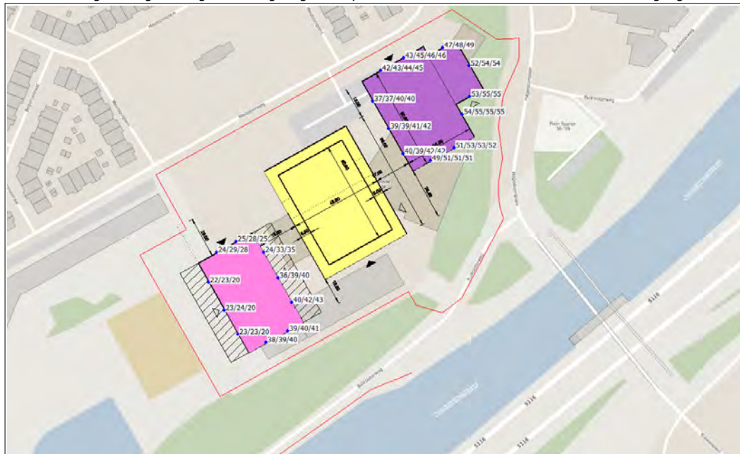
f3 Geluidbelasting vanwege de Hagedoornweg/Hagedoornplein (in dB Lden inclusief aftrek conform art. 110g Wgh).
