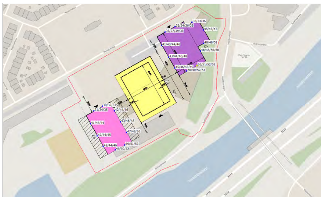
f2 Geluidbelasting vanwege de S116 (in dB Lden inclusief aftrek conform art. 110g Wgh).
