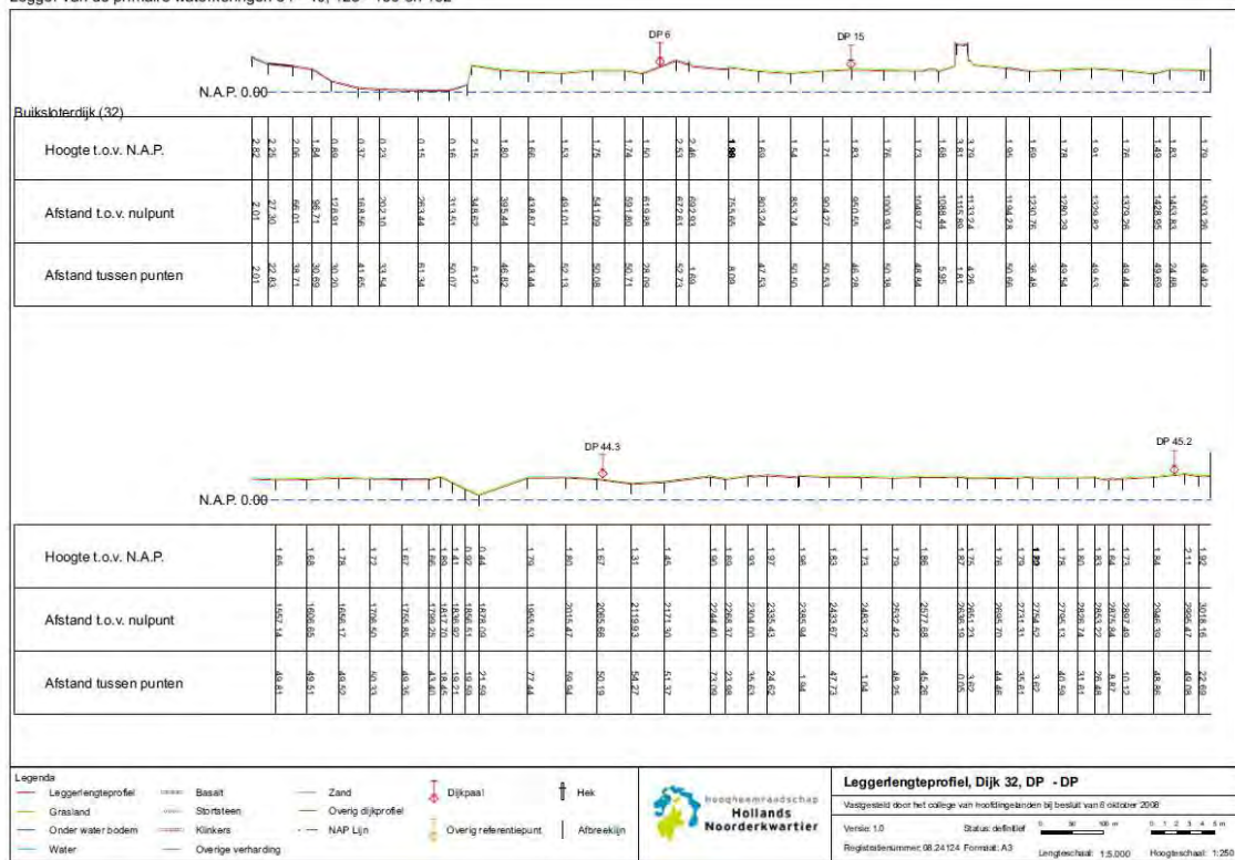
Figuur B-2 Lengteprofiel van dijk 32 [23][14].
