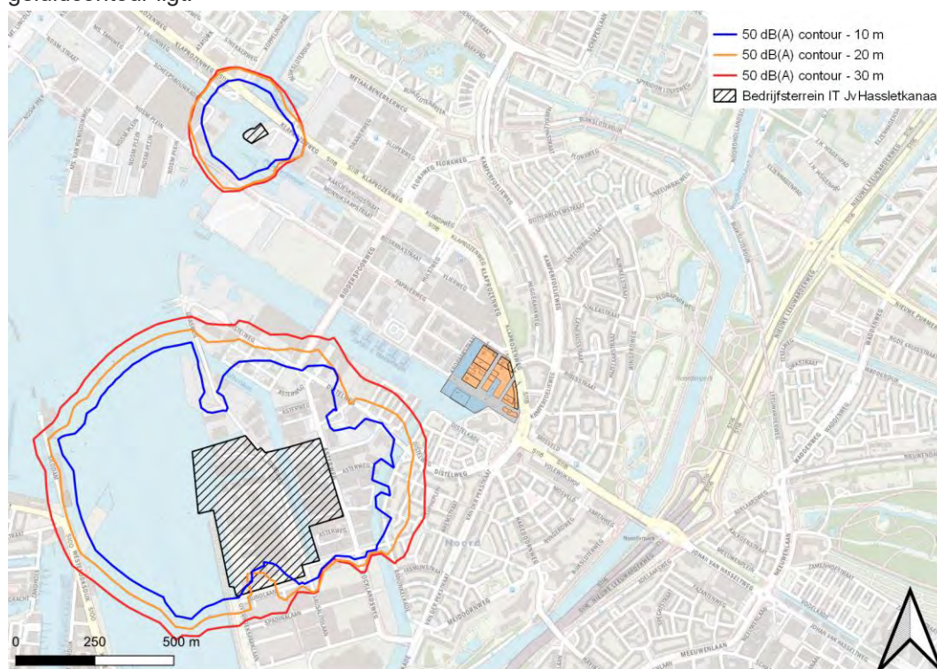
Figuur 2 50 dB(A)-geluidcontouren gezoneerd industrieterrein J. van Hasseltkanaal
