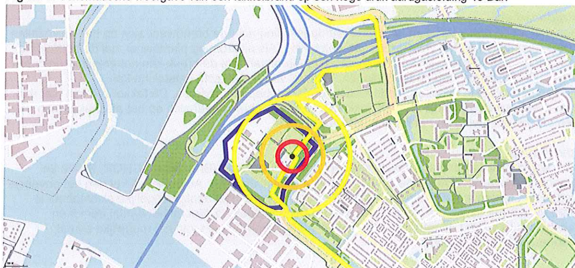
Figuur 4. Schematische weergave van een fakkelbrand op een hoge druk aardgasleiding 40 Bar.
