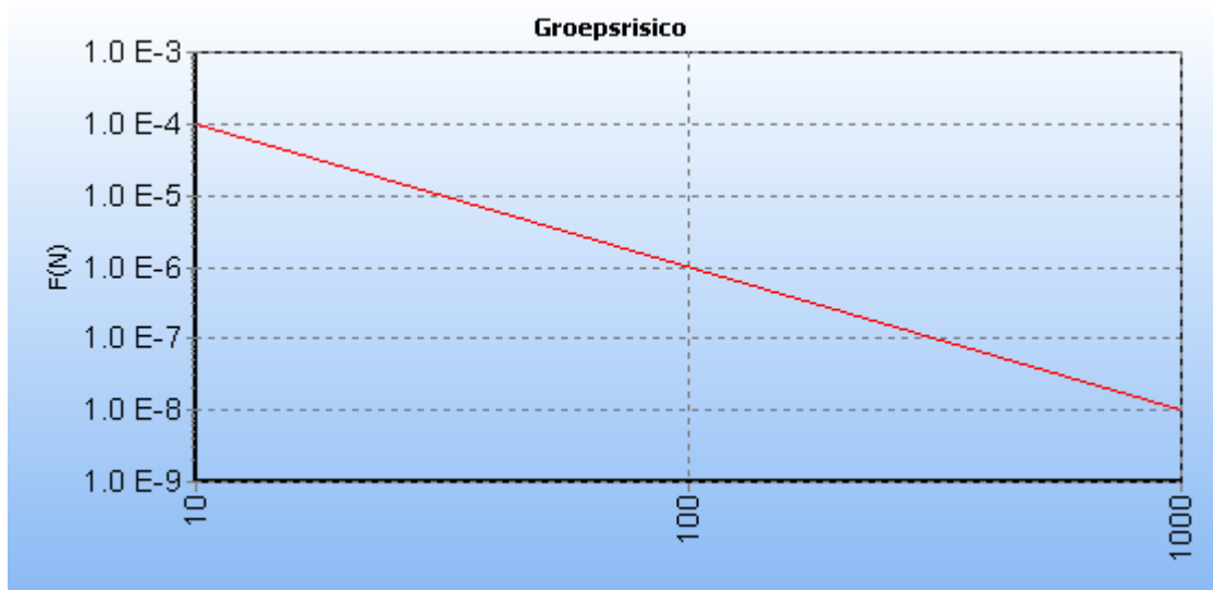
5.4 Figuur 5.4 FN curve voor W-572-13 van N.V. Nederlandse Gasunie voor de kilometer tussen stationing 0.00 en stationing 0.00
