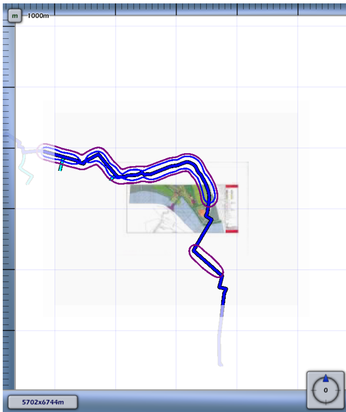
3.1 Figuur 3.1 Plaatsgebonden risico voor W-572-01 van N.V. Nederlandse Gasunie
