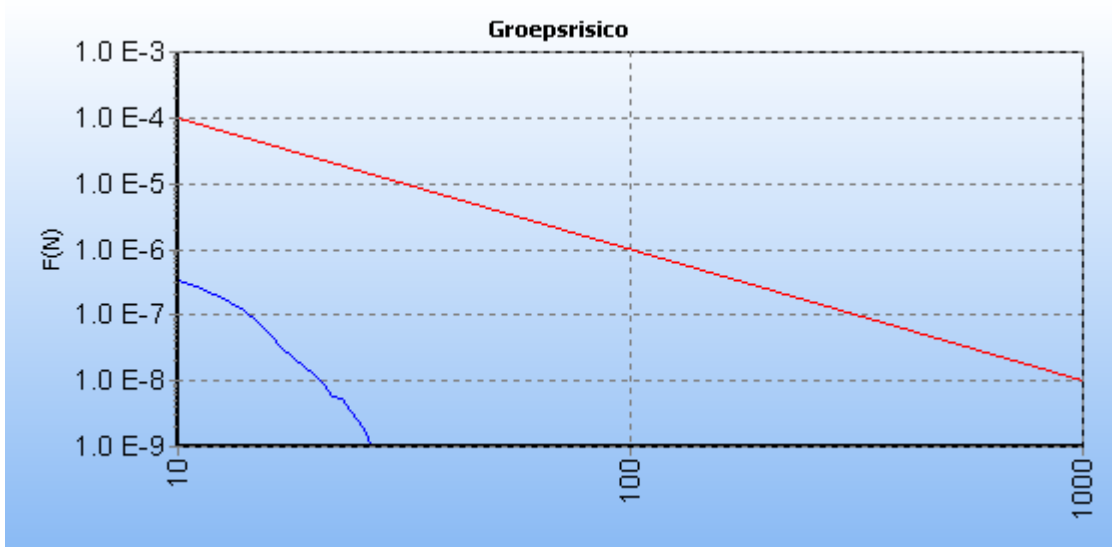
5.2 Figuur 5.2 FN curve voor W-572-02 van N.V. Nederlandse Gasunie voor de kilometer tussen stationing 0.00 en stationing 230.00
