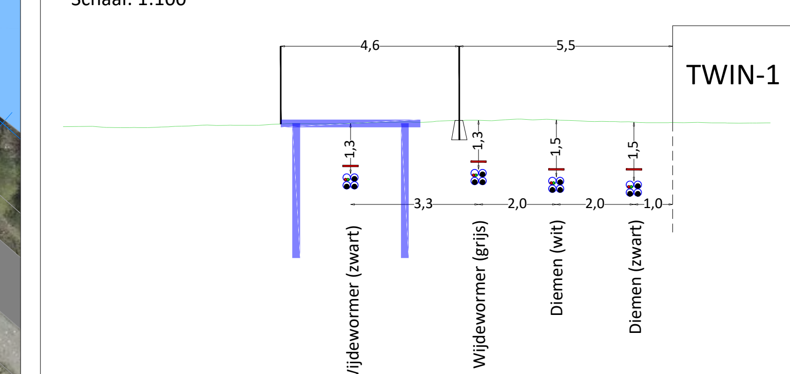
Doorsnede B-B Schaal: 1:100
