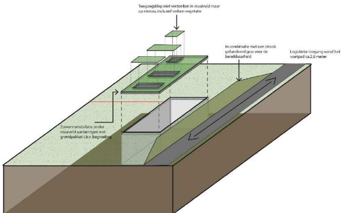
Afbeelding 2. Principeschets ondergrondse waterzuivering.
