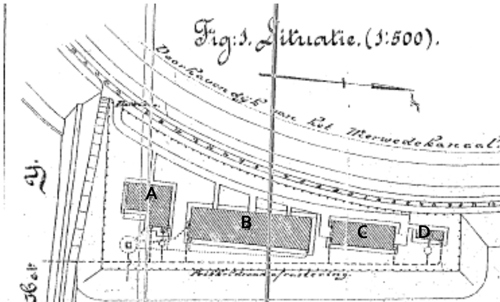
Uitsnede ontwerp-tekening voor het schiet- en exercitieterrein 1907. De tekening is west gericht. Figuur 1 toont situatietekening met vlnr: A. wachterswoning, B. schuilloods, C. schijvenloods en D. privaatgebouw. (Nationaal Archief).
