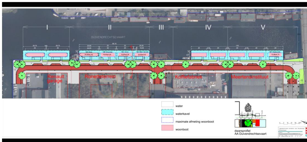
Figuur 1: Inrichtingsplan uit het Voorlopig ontwerp ontwerp integrale inrichting kade en ligplaatsen Duivendrechtse vaart / Joan Muyskenweg
