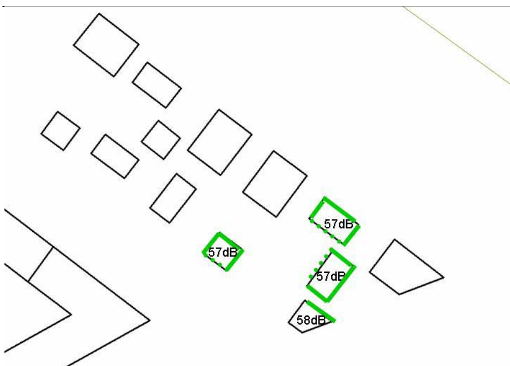
Figuur 5.4 Maximale geluidsbelasting losse bouwblokken zuid (groen = geluidsluwegevel, stippellijn = geluidsluwegevel op begane grond en 1e verdieping)
