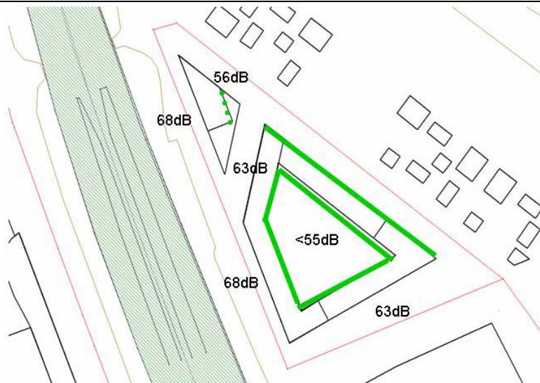
Figuur 6.2 Maximale geluidsbelasting Stadsblok met 2.1 meter scherm
