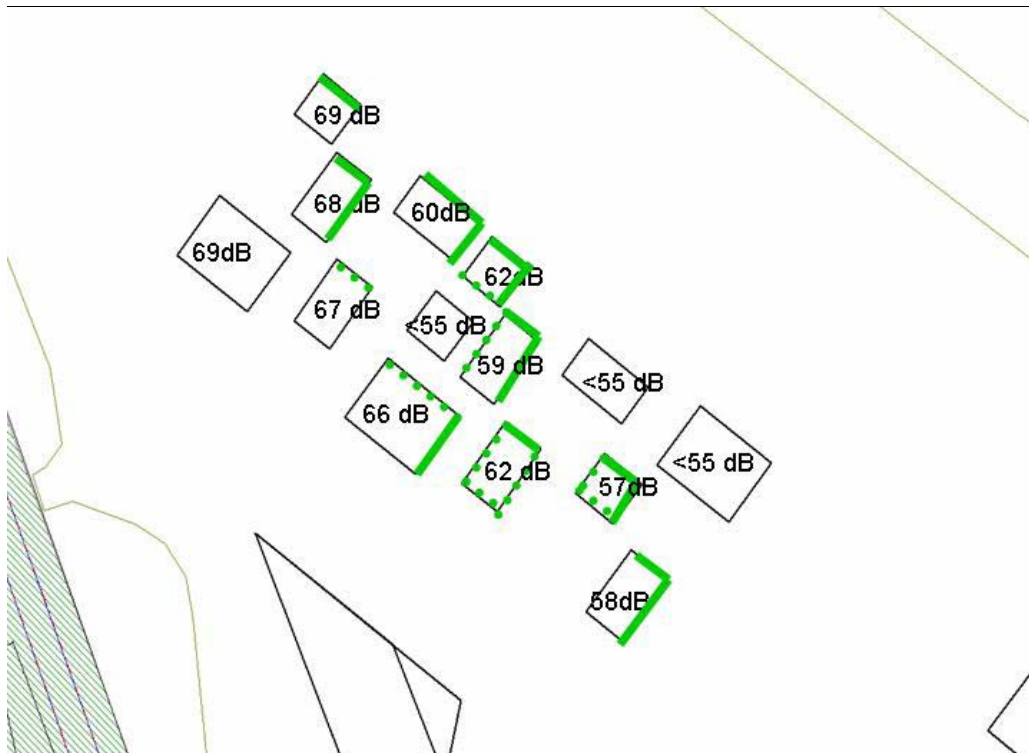
Figuur 5.3 maximale geluidsbelasting railverkeer losse bouwblokken noord (groen =geluidsluwegevel, stippelijn = geluidsluwegevel op begane grond en 1e verdieping)
