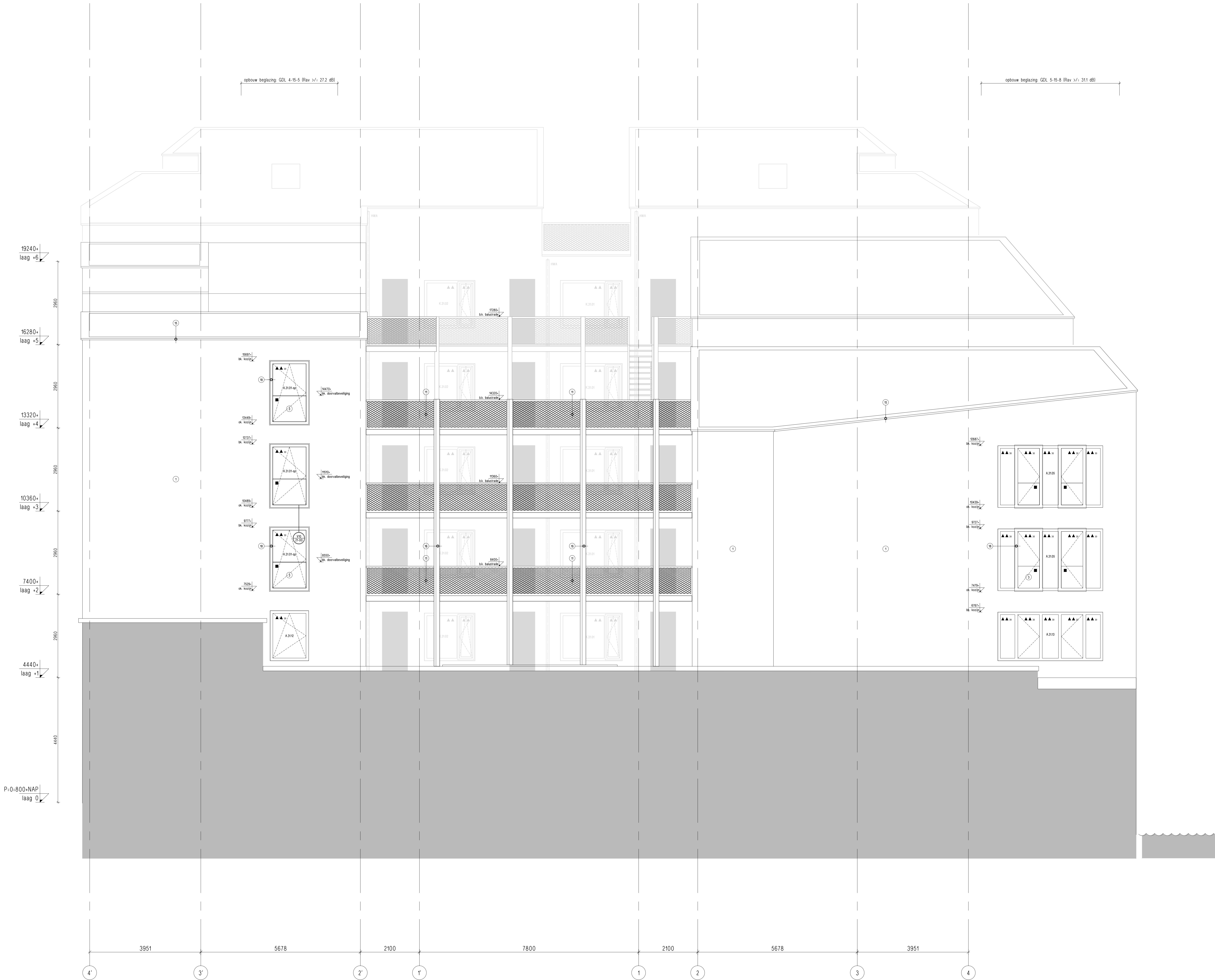
WESTGEVEL
