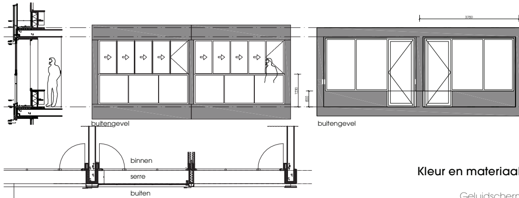
■ dubbele gevel
