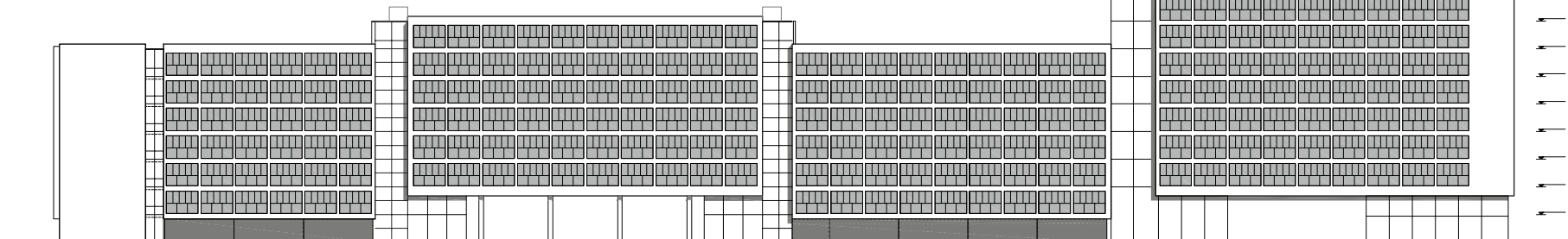
■ gevel spoorzijde
