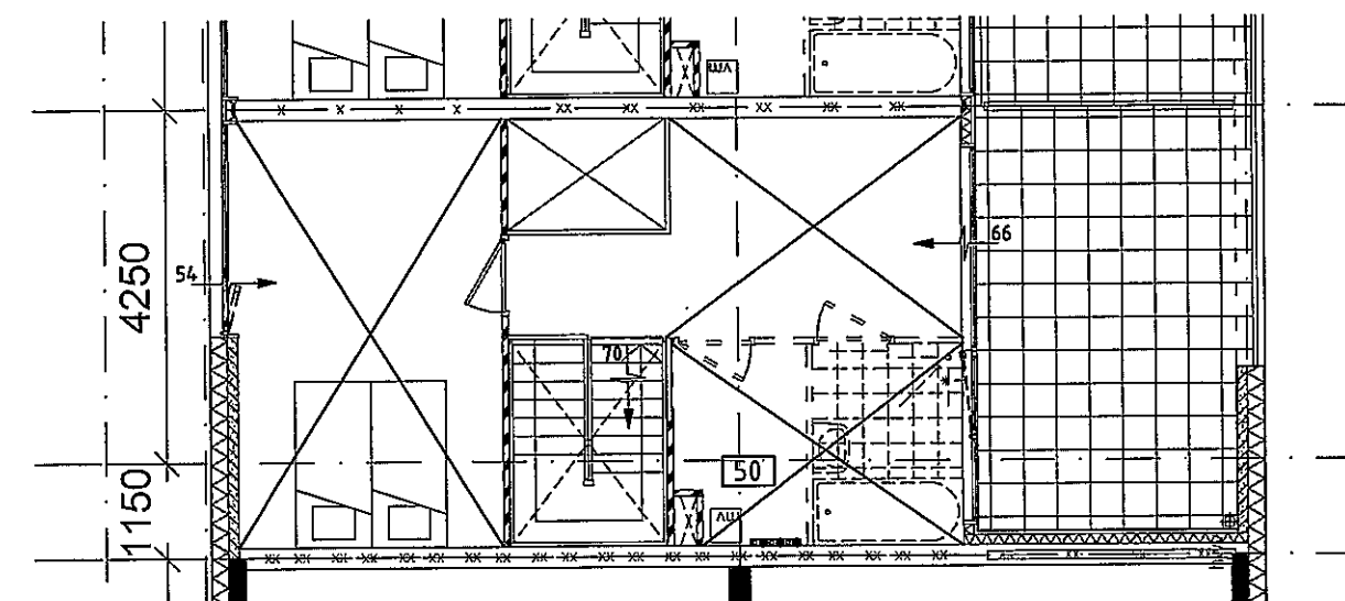
2e verdieping
