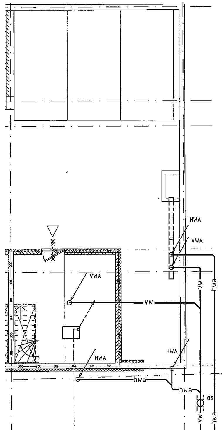
kelder
