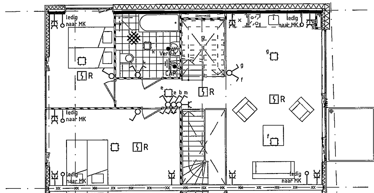
1e verdieping
