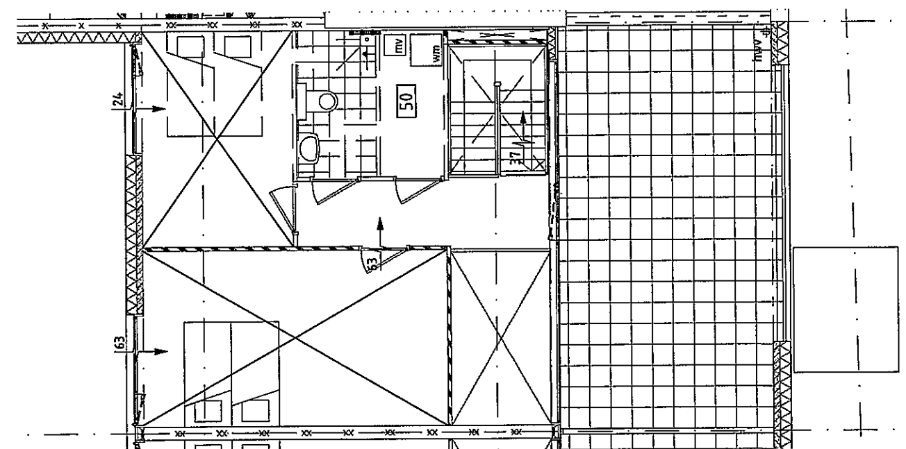
2e verdieping
