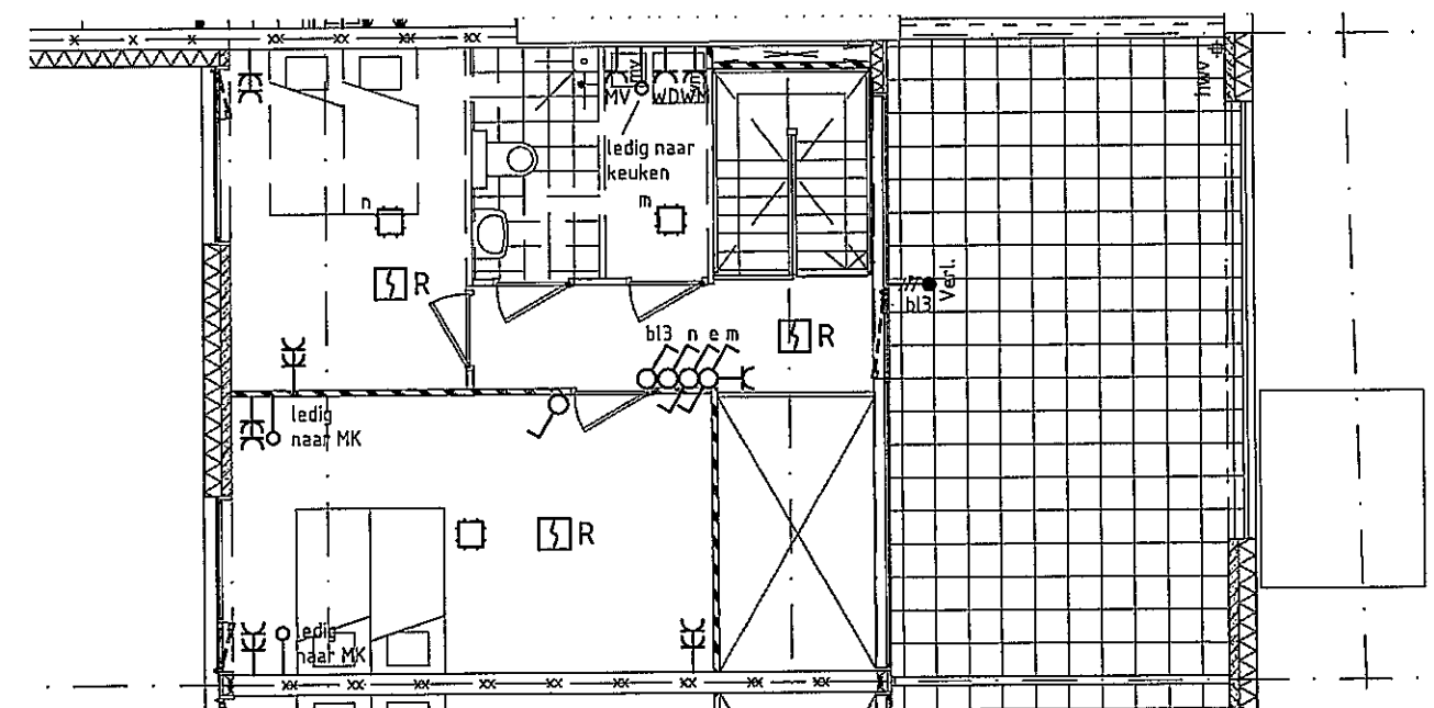
2e verdieping
