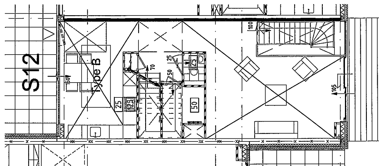
begane grond
