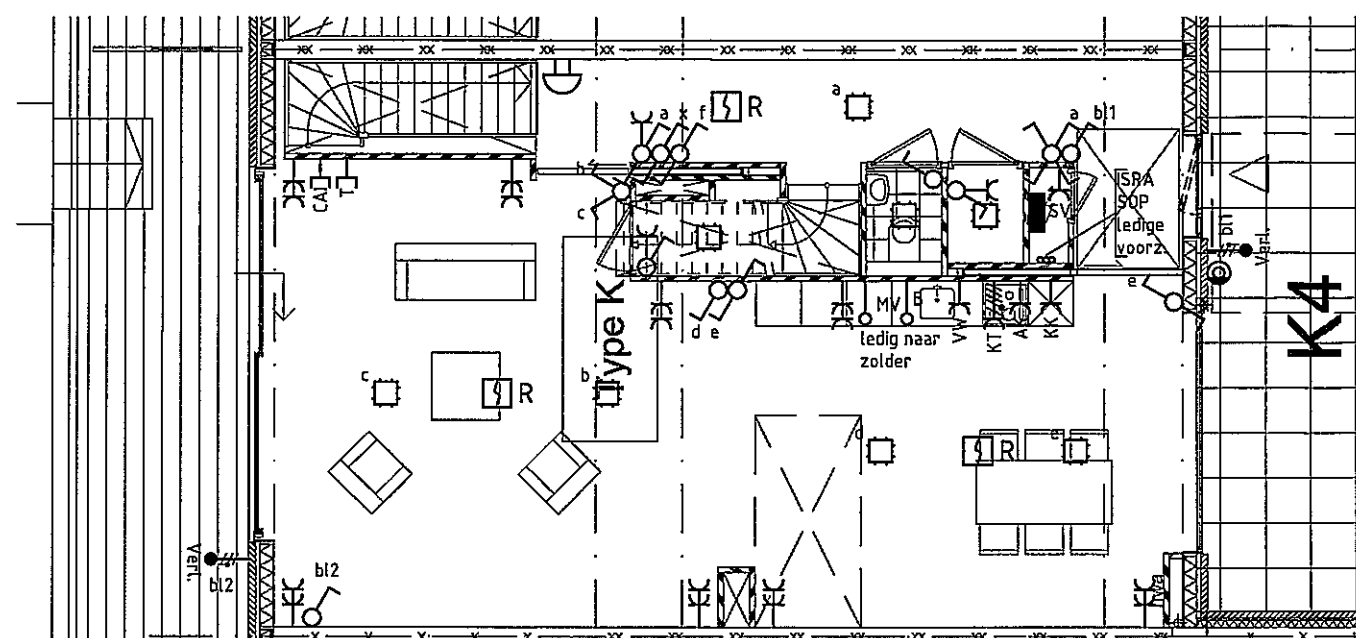
begane grond
