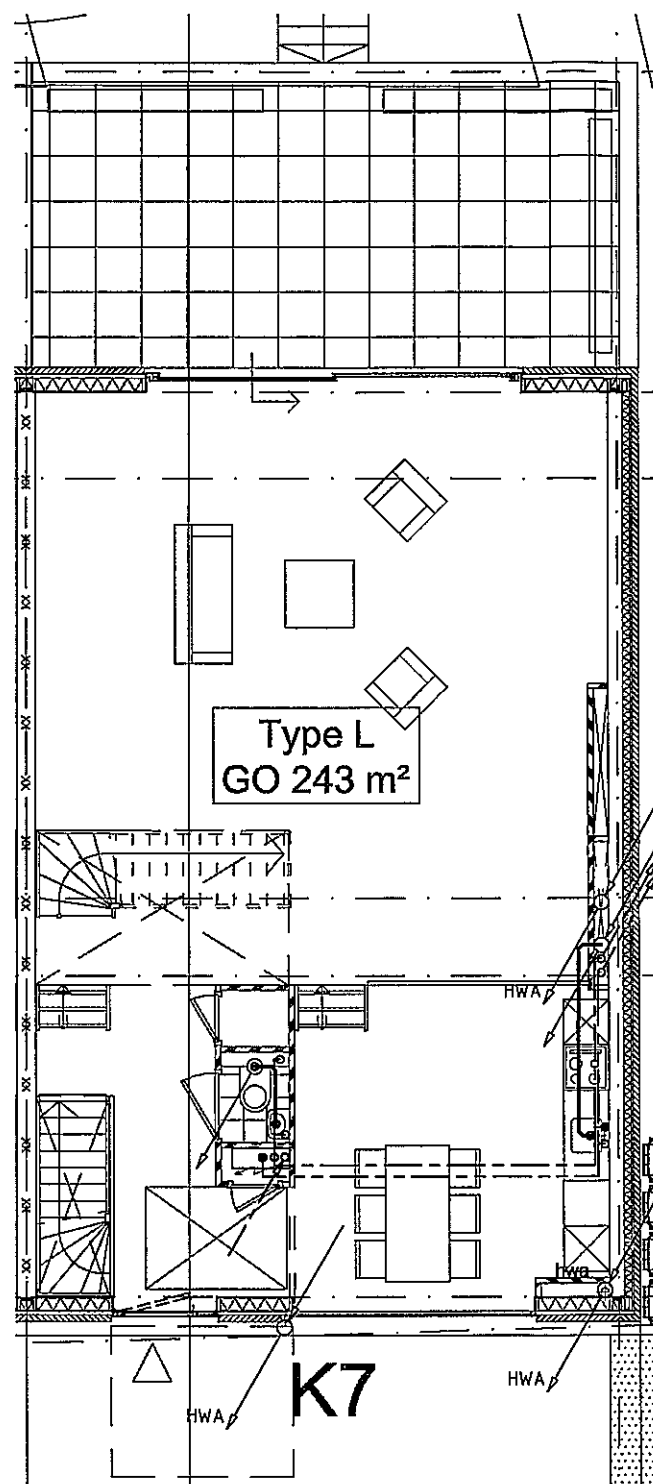
begane grond
