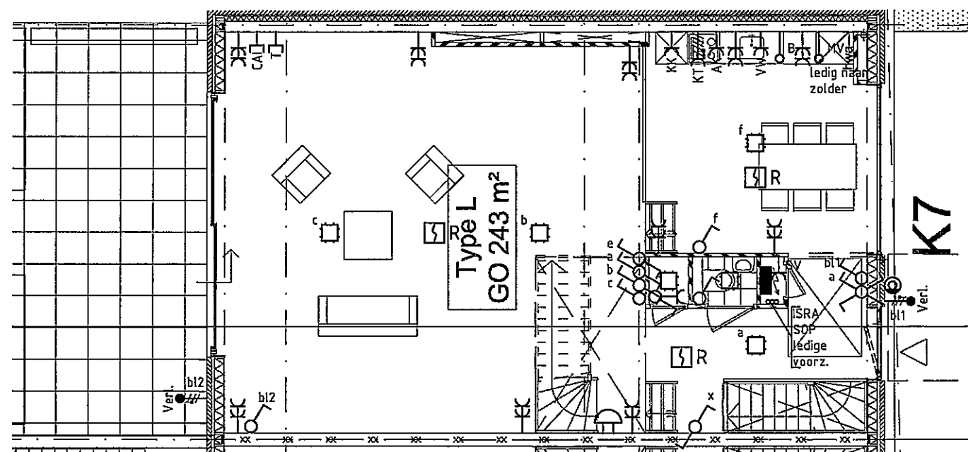
begane grond
