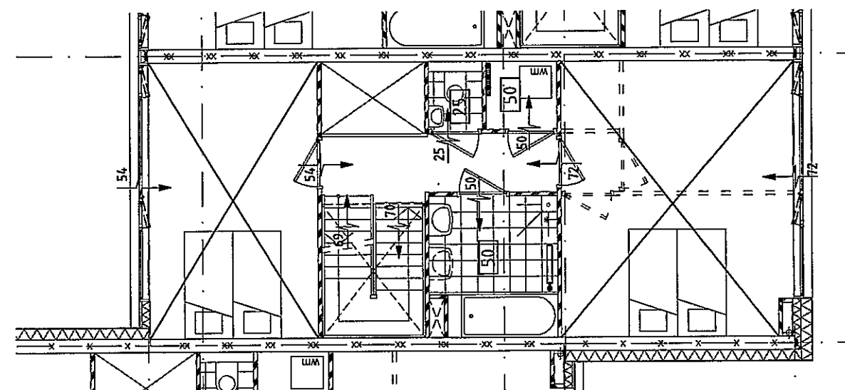
1e verdieping
