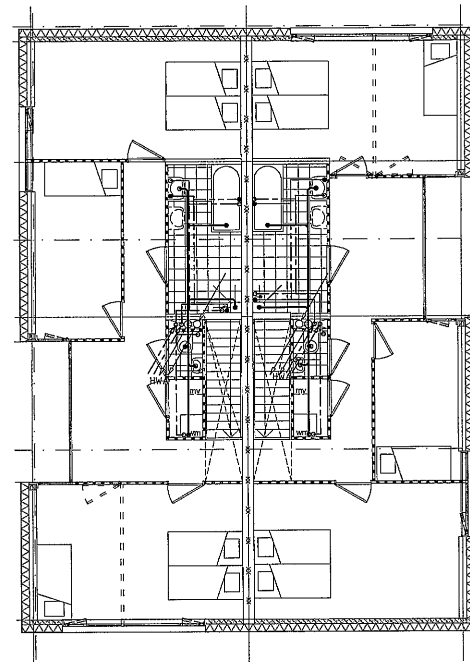
2e verdieping
