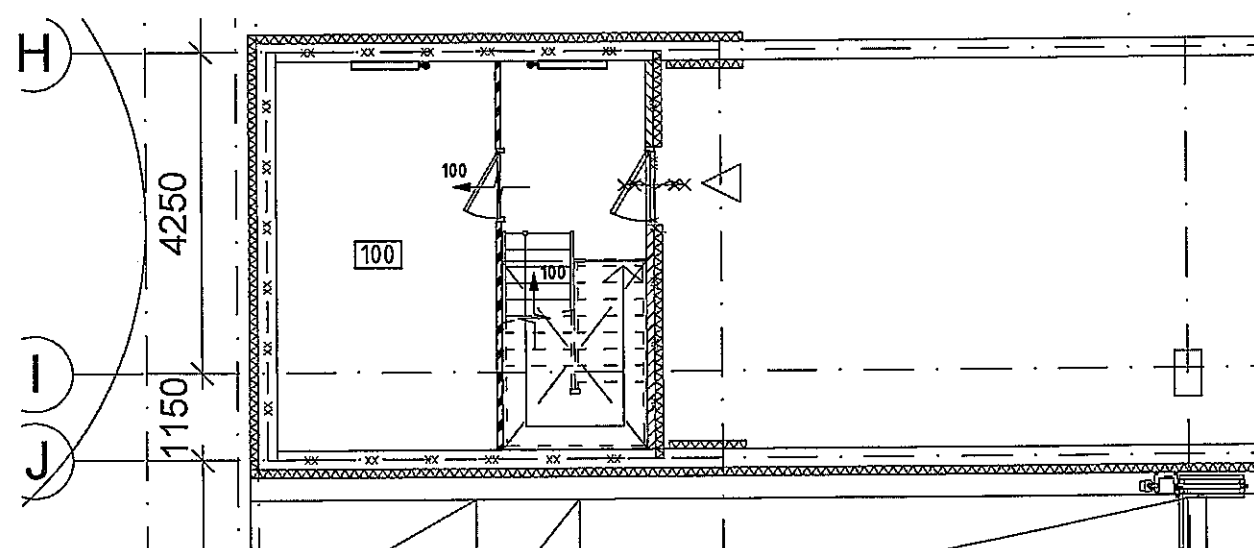
kelder
