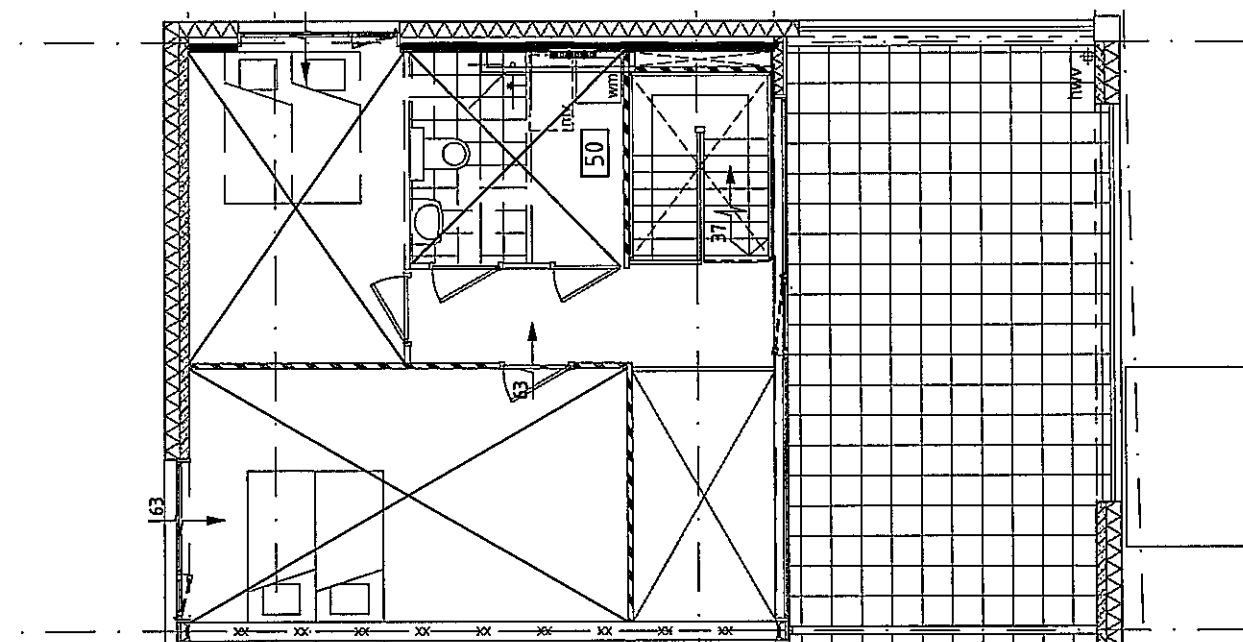
2e verdieping
