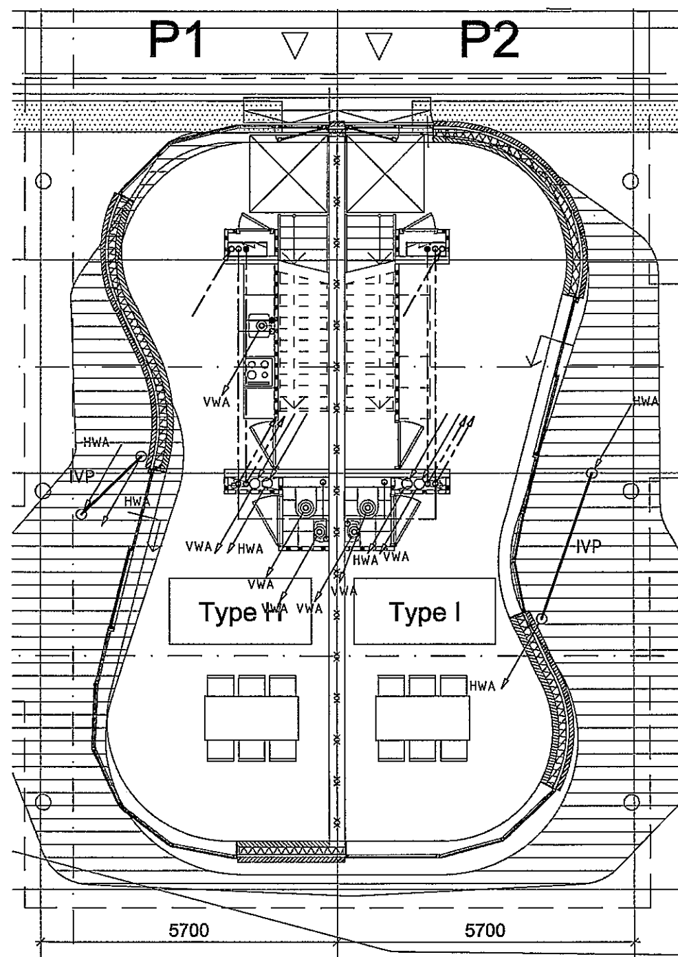
begane grond
