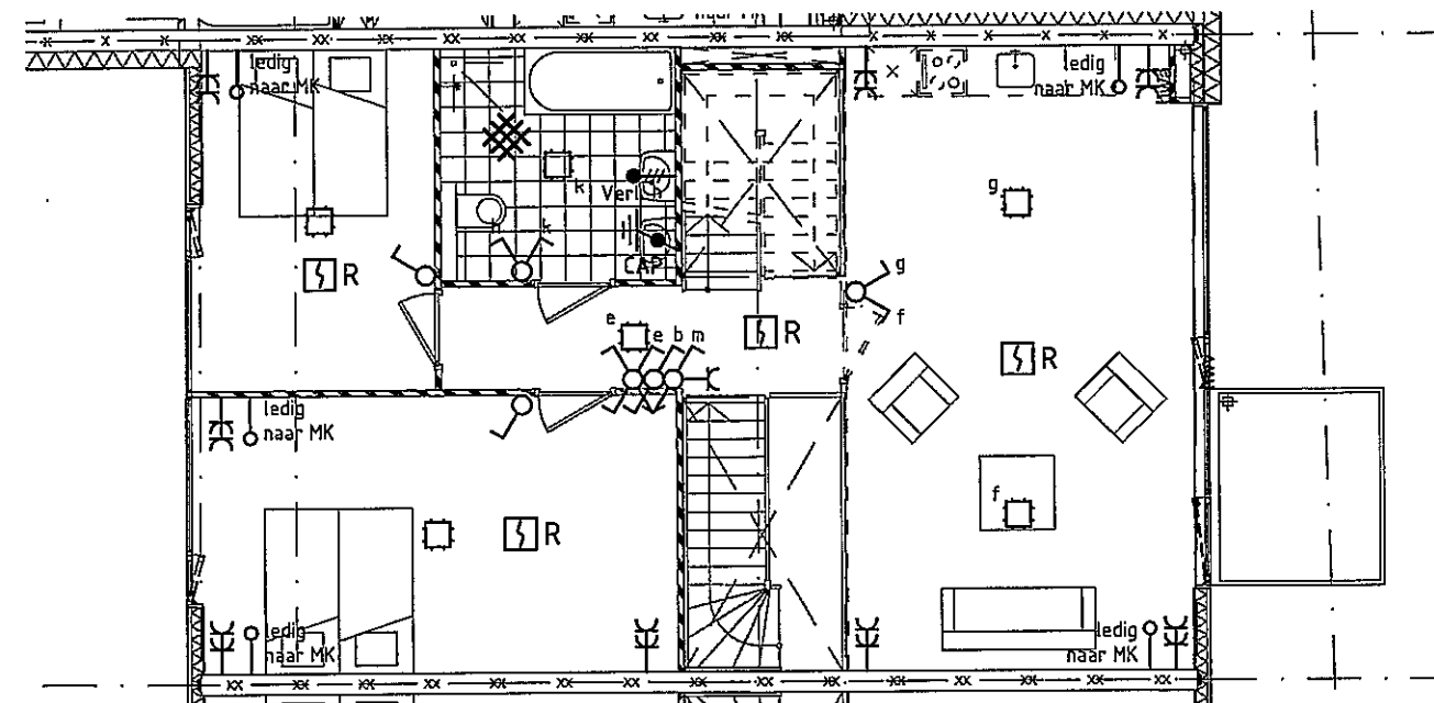
1e verdieping
