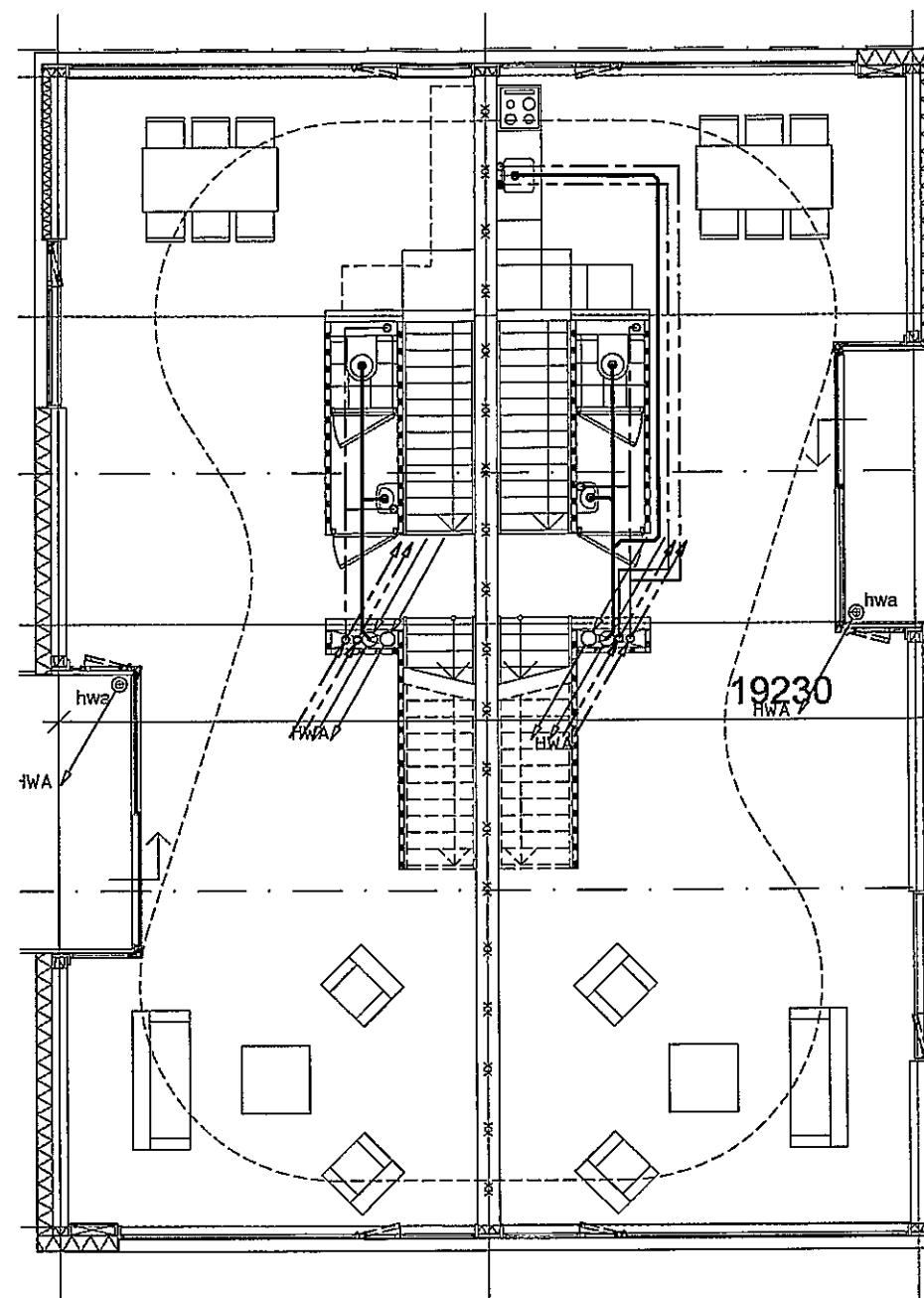
1e verdieping
