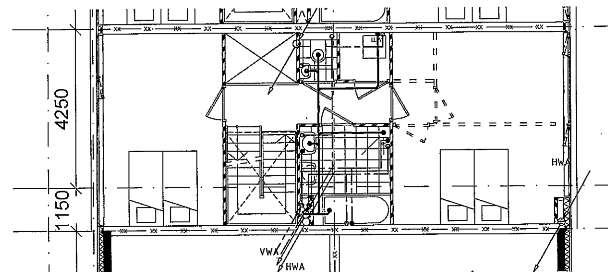
1e verdieping
