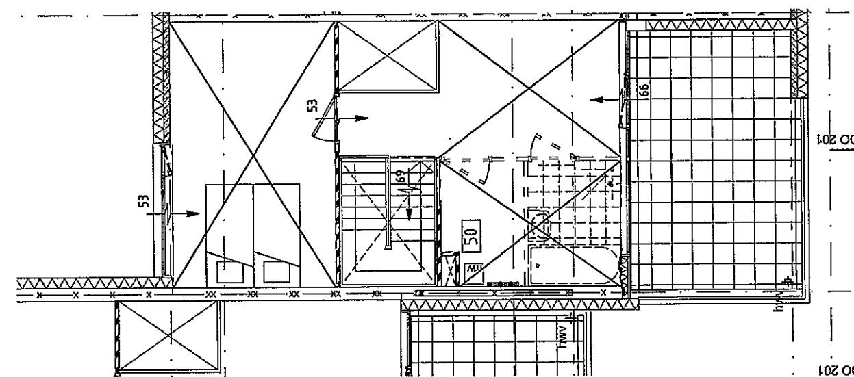
2e verdieping
