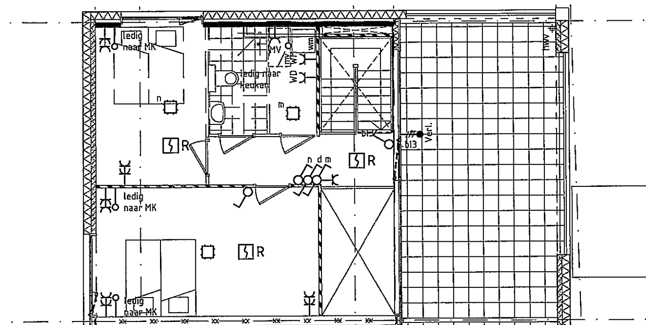
2e verdieping
