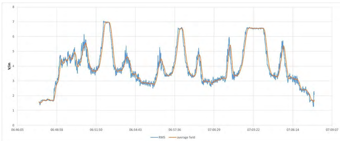
Figuur A3 Elektrische veldsterkte als functie van de tijd (meetpunten 5, 6 en 7).
