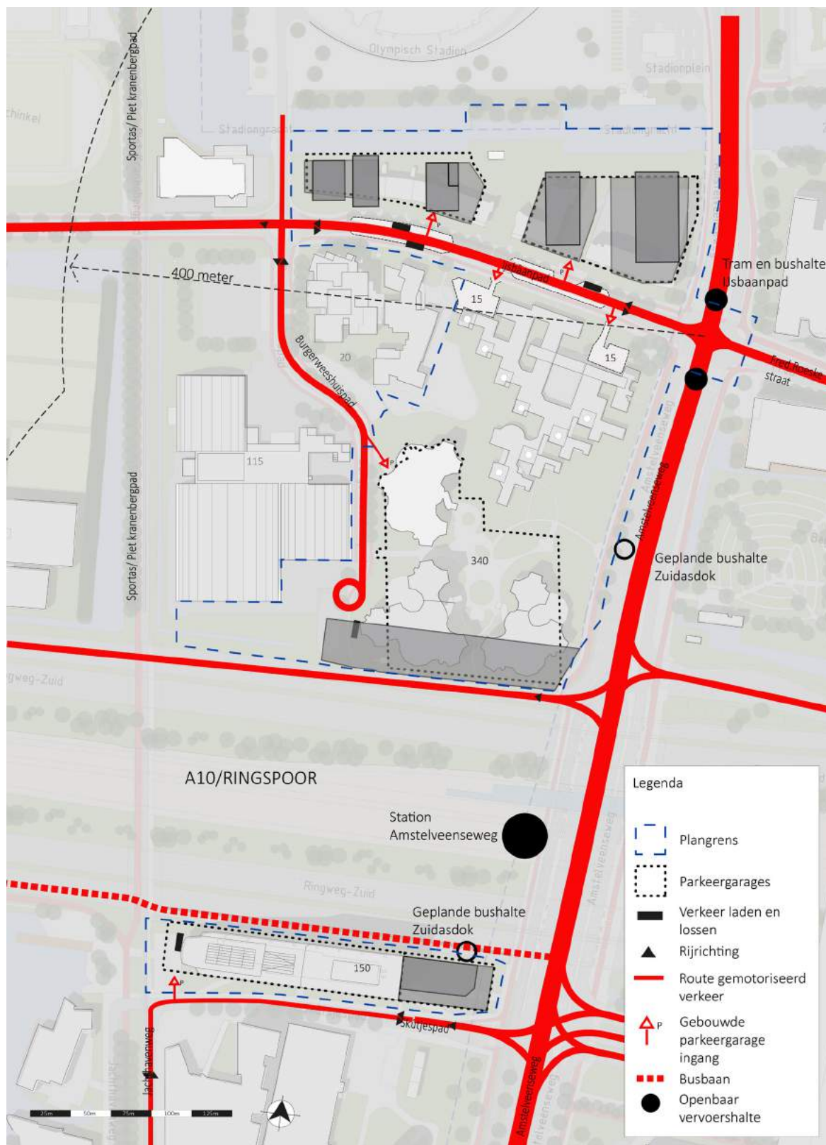
Figuur 19: ontsluiting gemotoriseerd verkeer, parkeergarages en laden en lossen
