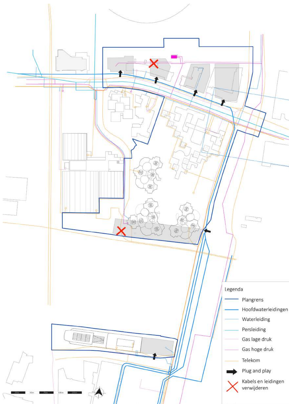
Figuur26: huidige kables en leidingen met ontwikkelvelden
