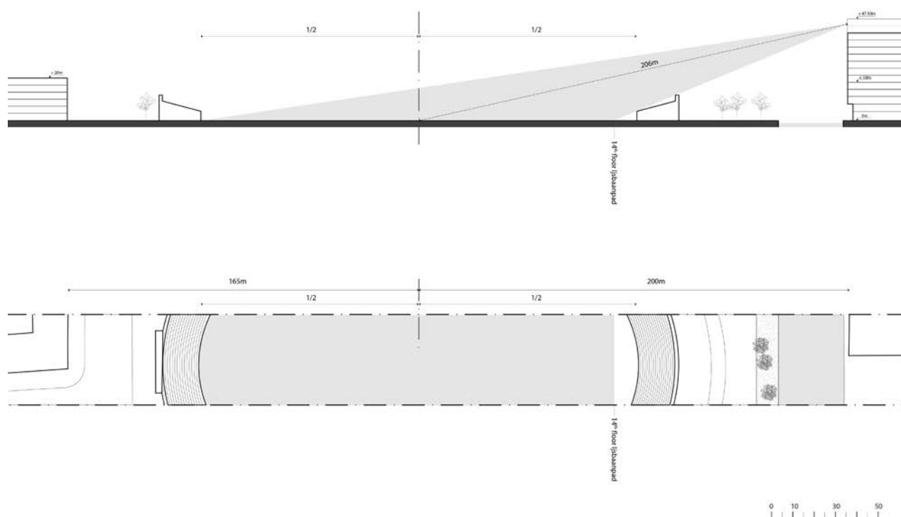
Figuur 1: zichtlijn vanuit de hoogste verdieping van het toekomstige gebouw aan het Noordzone IJsbaanpad
