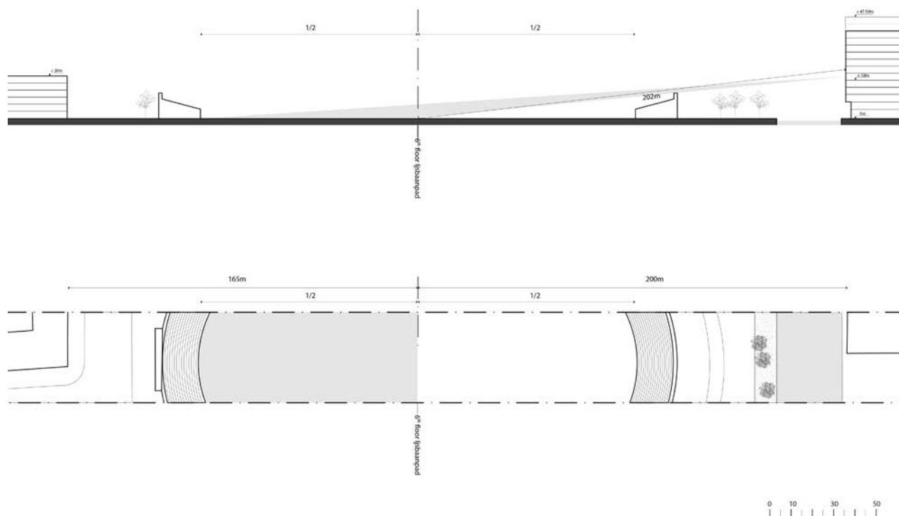
Figuur 2: zichtlijn vanuit de 6 e verdieping van het toekomstige gebouw aan het Noordzone IJsbaanpad
