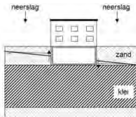
Figuur 3: schematische weergave van barrièrewerking (bron Fugro)
