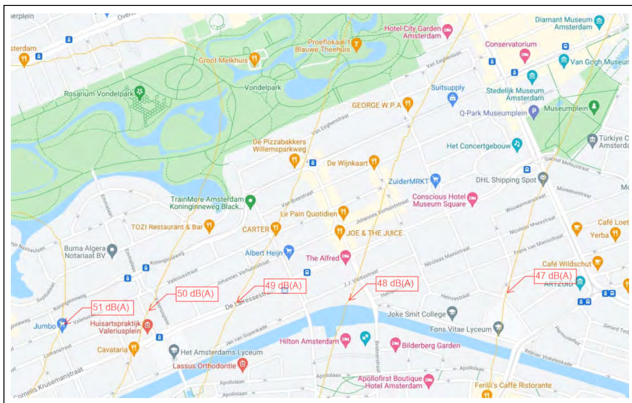
Figuur 3.1: Geluidbelastingen luchtvaartlawaai Schiphol
