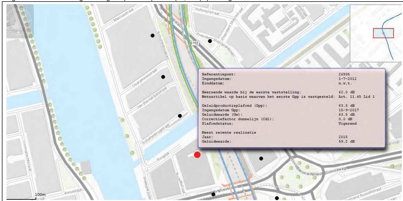
Figuur 2.1: Maatgevende geluidproductieplafond (63,5 dB) spoorweglawaai
