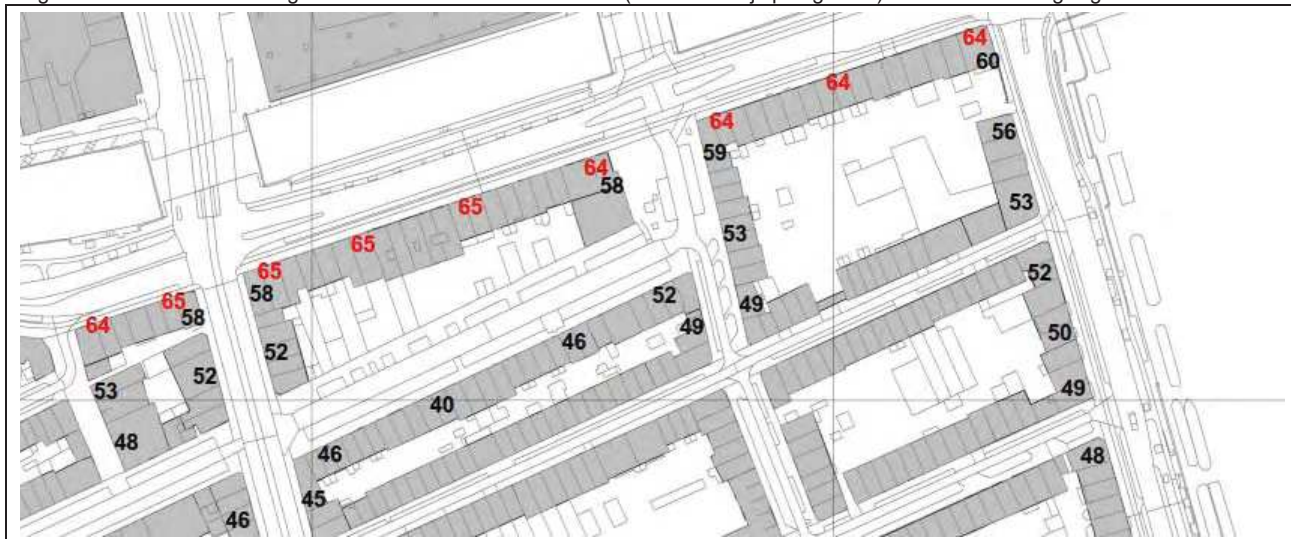
Figuur 5.10: Geluidbelastingen Stadhouderskade/Mauritskade (Noordoostelijk plangebied) na aftrek art. 110g Wgh.
