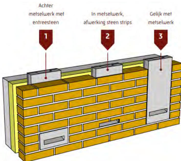
Figuur 4. Voorbeeld van een kast voor een zomer- of paarverblijfplaats van Unitura (Vleermuiskast VMPPM1)
